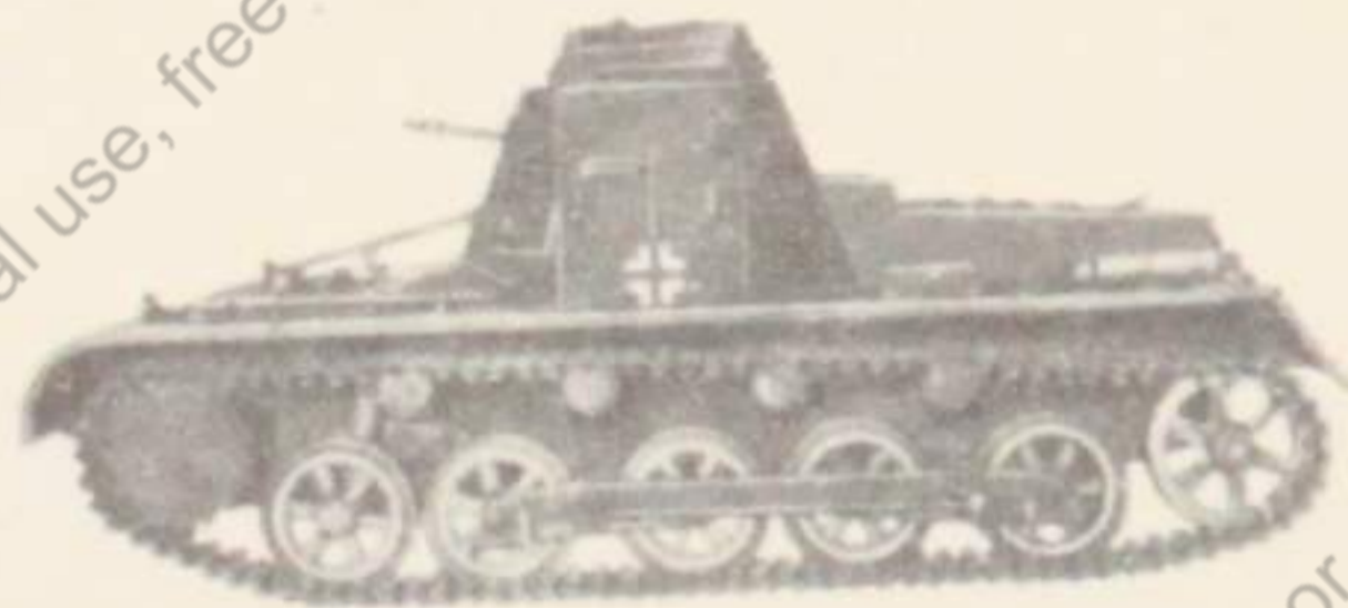
kleiner Panzerbefehlswagen
