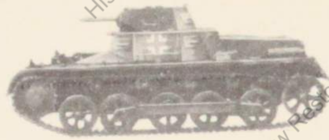
Panzerkampfwagen I
