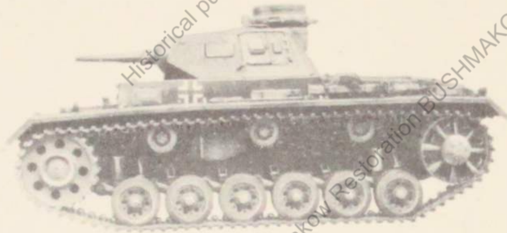
Panzerkampfwagen III
