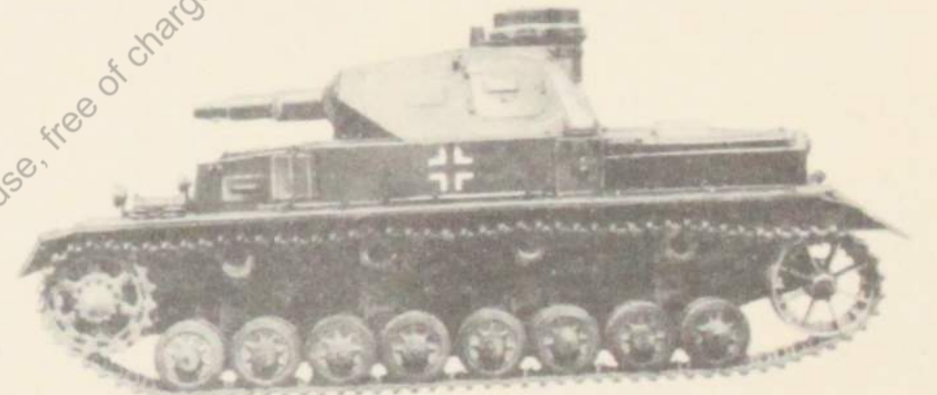
Panzerkampfwagen IV
