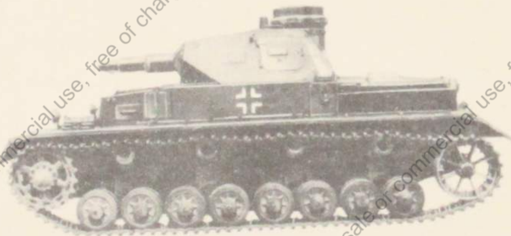
Panzerkampfwagen IV
