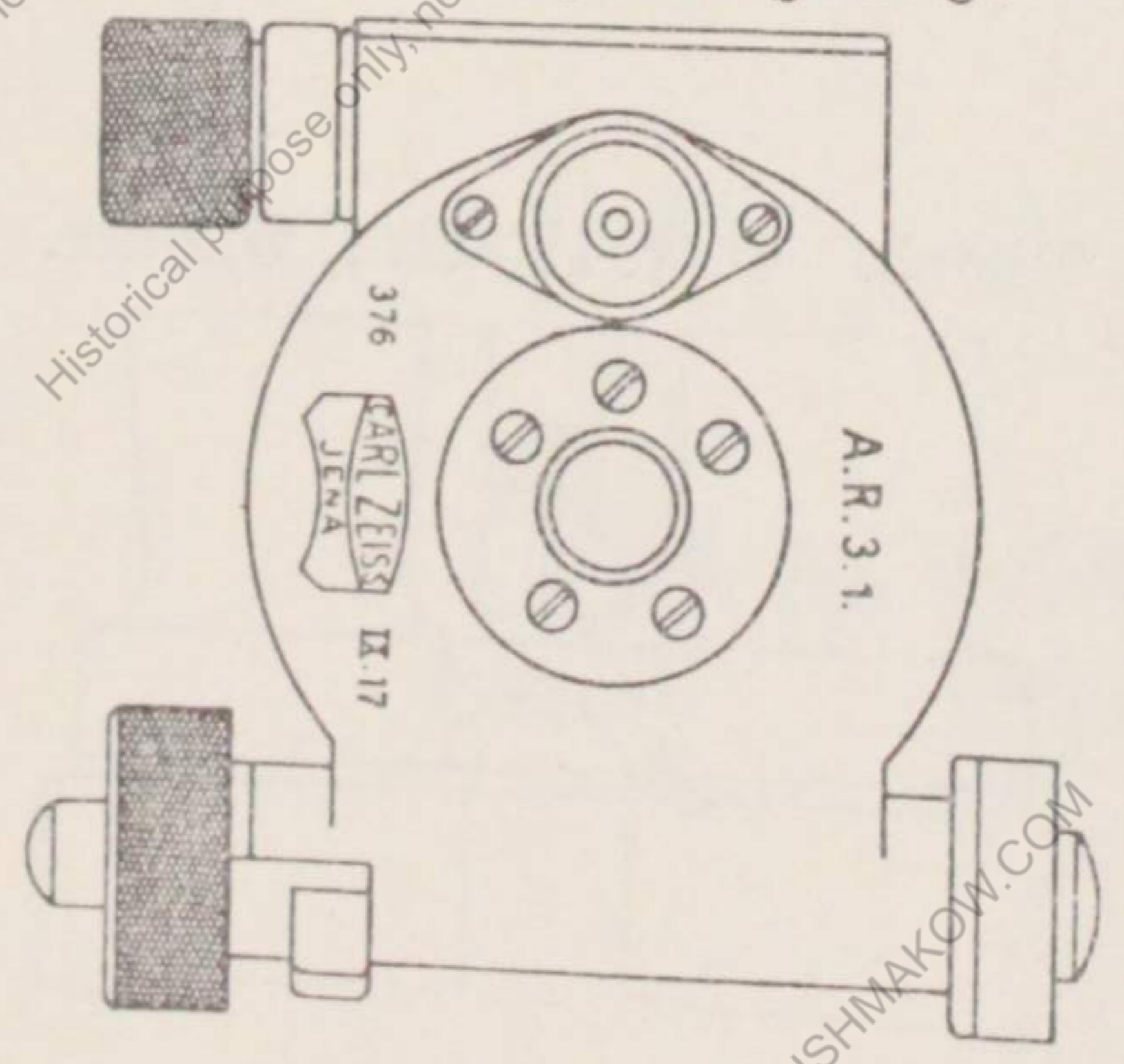
Bild 6. Meßkreis 3. G. F.
