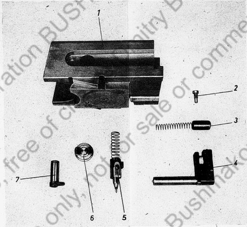
Einzelteile vom Verschußkeil
