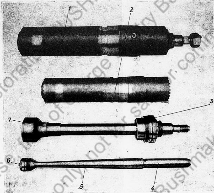
Rohrbremse
