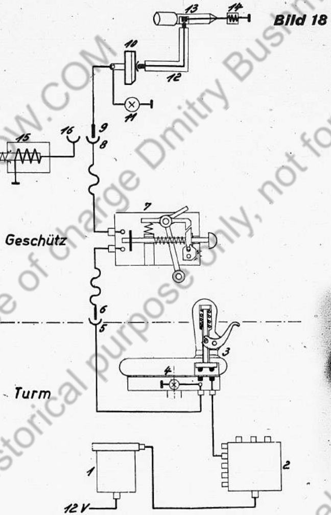
Leitungsplan der elektrischen Abfeuerung
