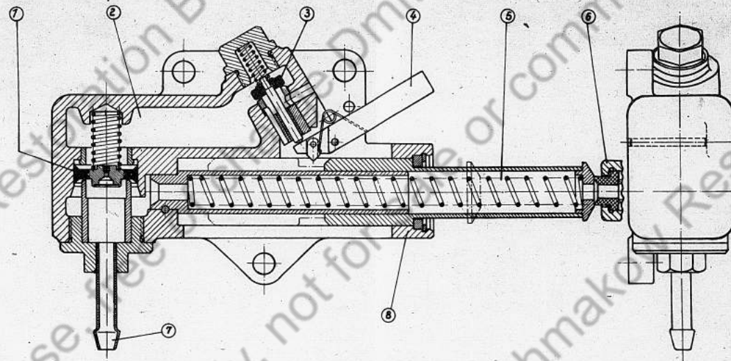
Ausblaseventil
