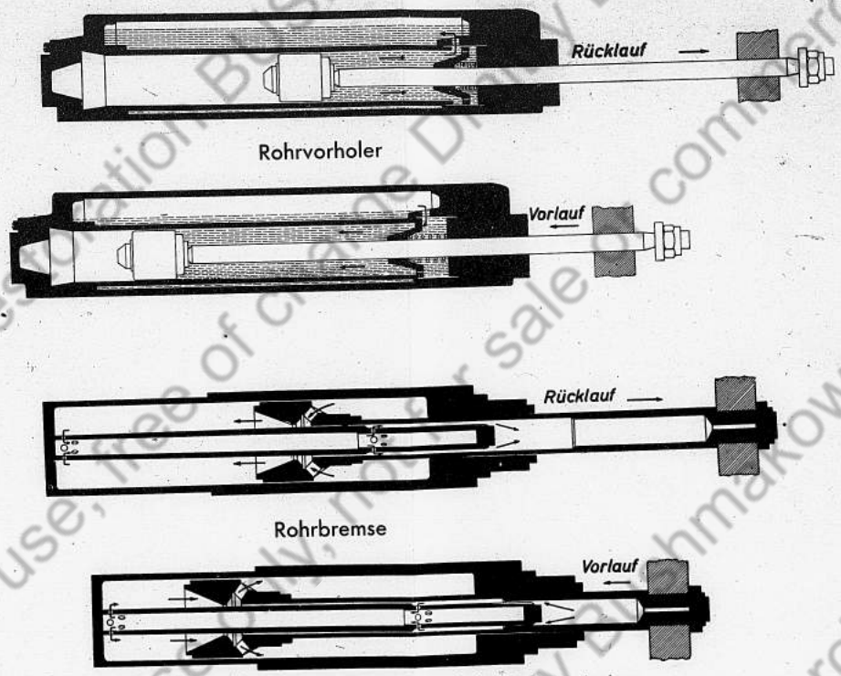
Wirkungsweise der Rohrbremse und des Rohrvorholers
