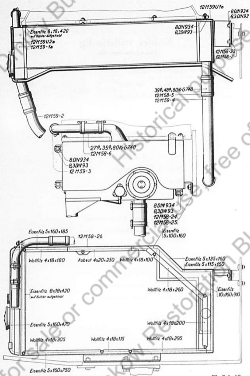
60 Gruppe 12 M 59a Kühler (Für 1. Hälfte 5. Serie) Tafel 46.
