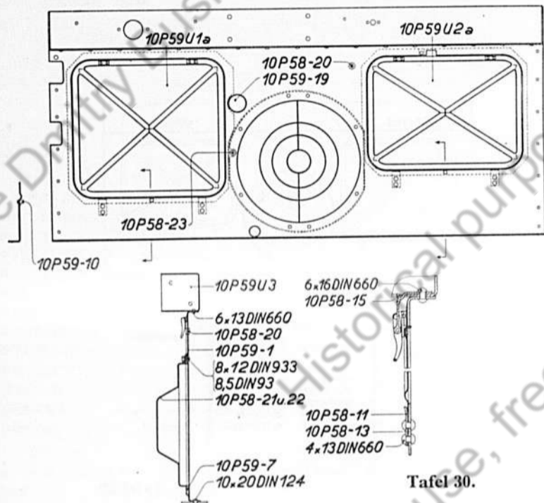
Zwischenwand, vollständig (Ab 6. Serie)
