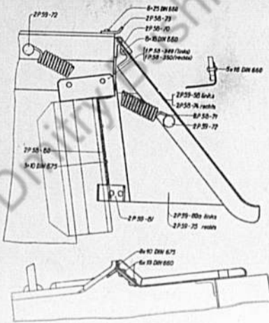
Hinterteil zur Kettenabdeckung
