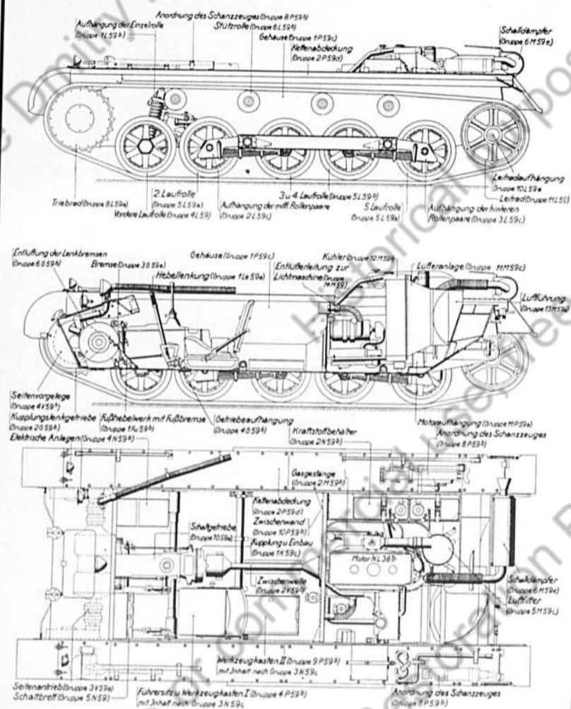
Zusammenstellung des Fahrgestells Tafel 1.
