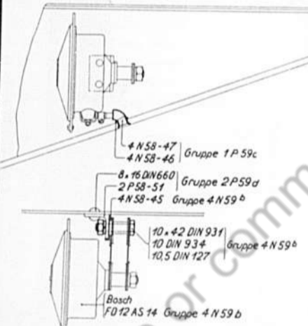
Befestigung des Boschhornes
