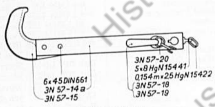
Kettenspanner
