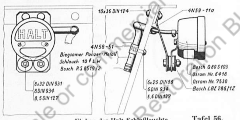
Einbau der Halt-Schlußleuchte Tafel 56.
