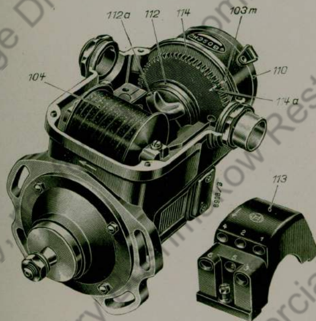
Abb. 12/2 Magnetzünder, Schutzkapsel und Verteilerbogen abgenommen
