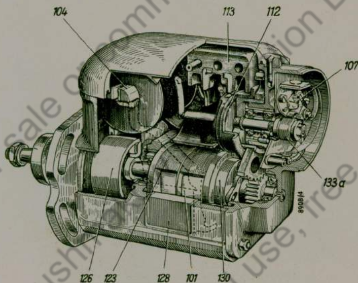
Abb. 12/1 Magnetzünder, aufgeschnitten
