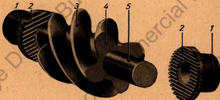
Schneckenrad-Ausgleichgetriebe, Sperrschnecke mit Bundbuchsen
