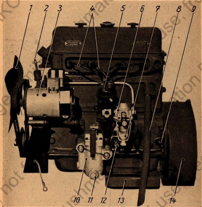
Motor, linke Seitenansicht, entfört nach Gruppe III
