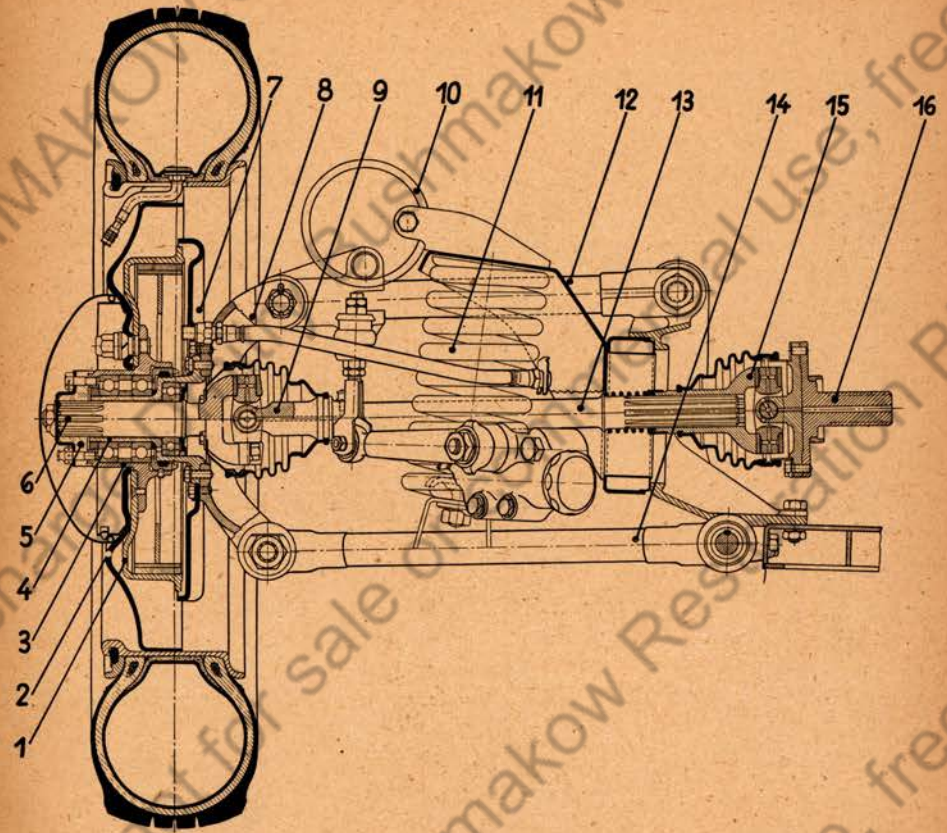
Hinterer Radantrieb, Schnitt
