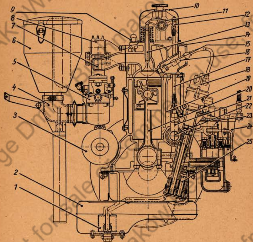
Motor, Querschnitt, entführt nach Gruppe III
