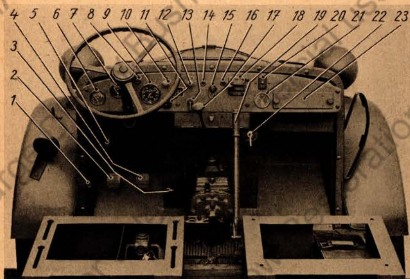
Hand- und Fußhebelwerk, Schaltbrett
