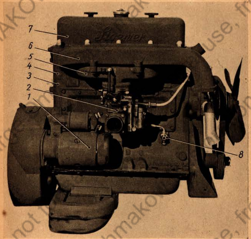
Motor, rechte Seitenansicht
