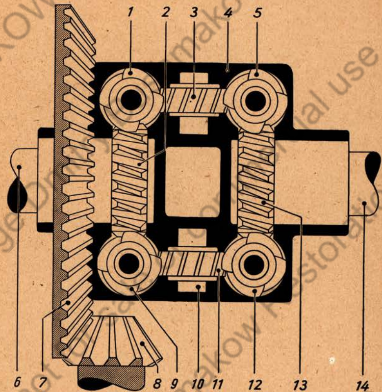
Schneckenrad-Ausgleichgetriebe (Schema)
