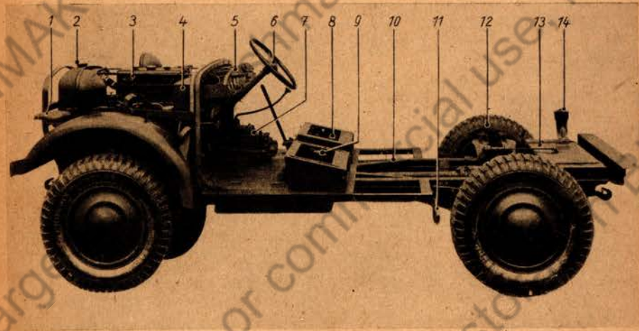
Fahrgerüst, Ansicht von links
