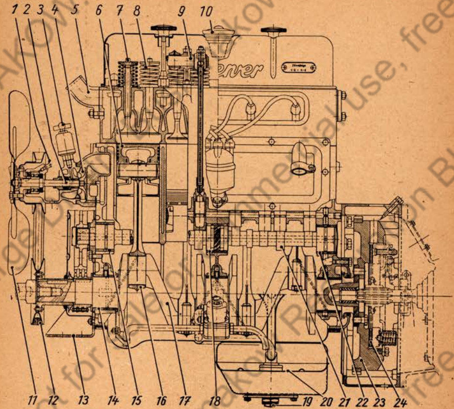
Motor, Längsschnitt
