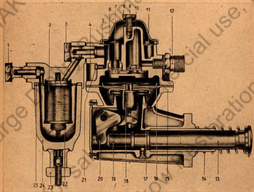
Kraftstoffpumpe mit Filter
