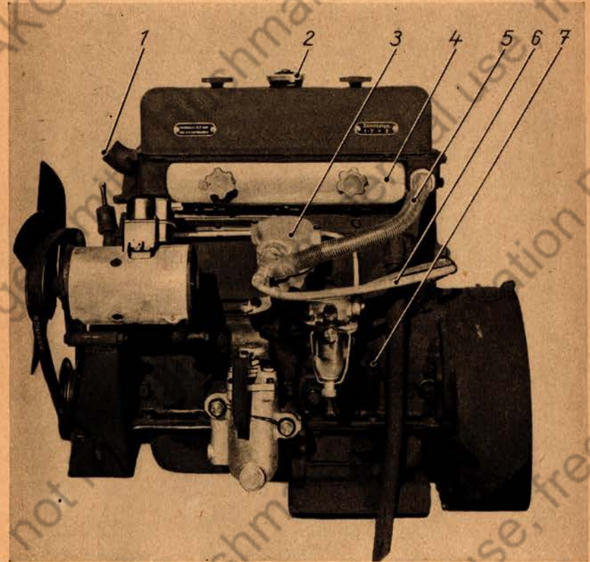
Motor, linke Seitenansicht, entört nach Gruppe 1
