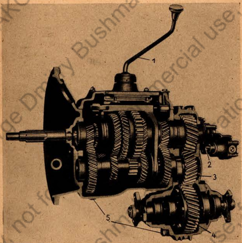
Wegfelgetriebe (5 Ganggetriebe)
