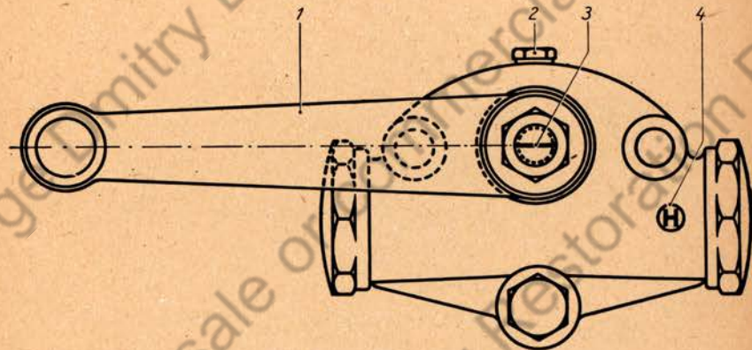
Stoßdämpfer (Sichtel & Sack's DUO 40 CK)
