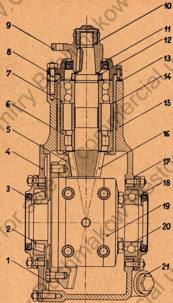
Achsantrieb, Schnitt
