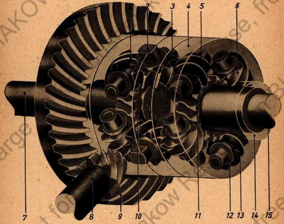
Schneckenrad-Ausgleichgetriebe, Gesamtansicht
