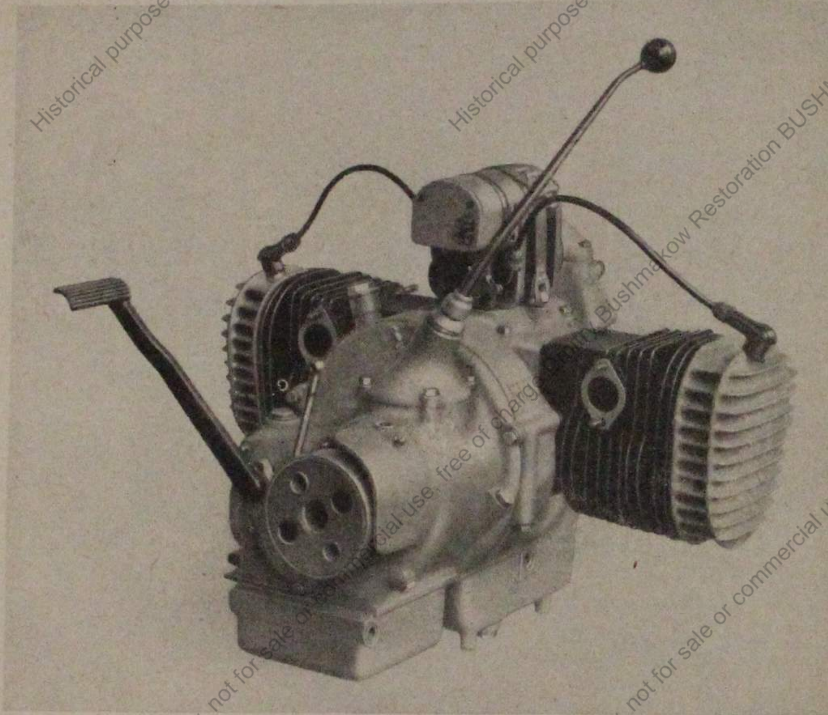
Tafel 1, Gruppe M: Motor und Getriebe
