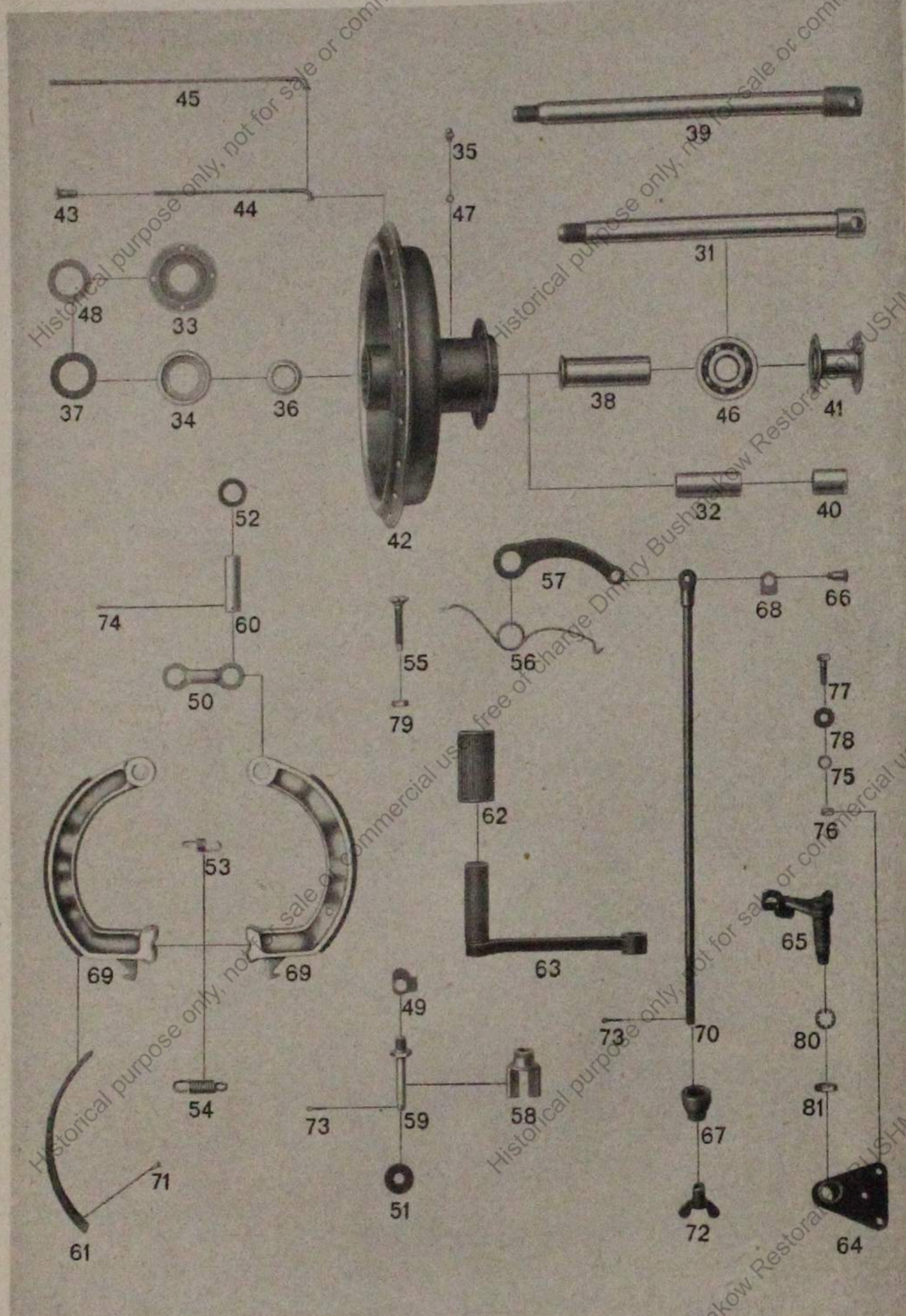
Tafel 23, Gruppe B: Räder und Bremsen
