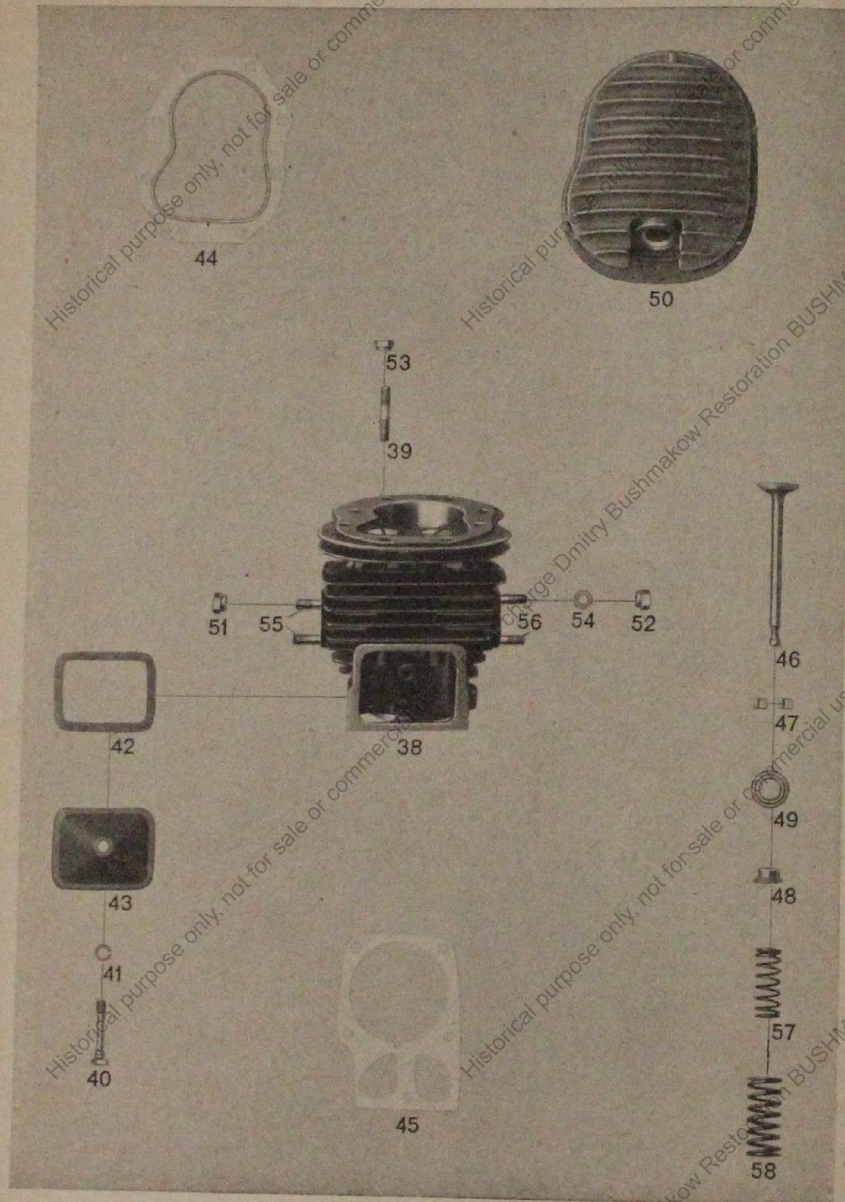
Tafel 3, Gruppe M: a) Motor, Zylinder
