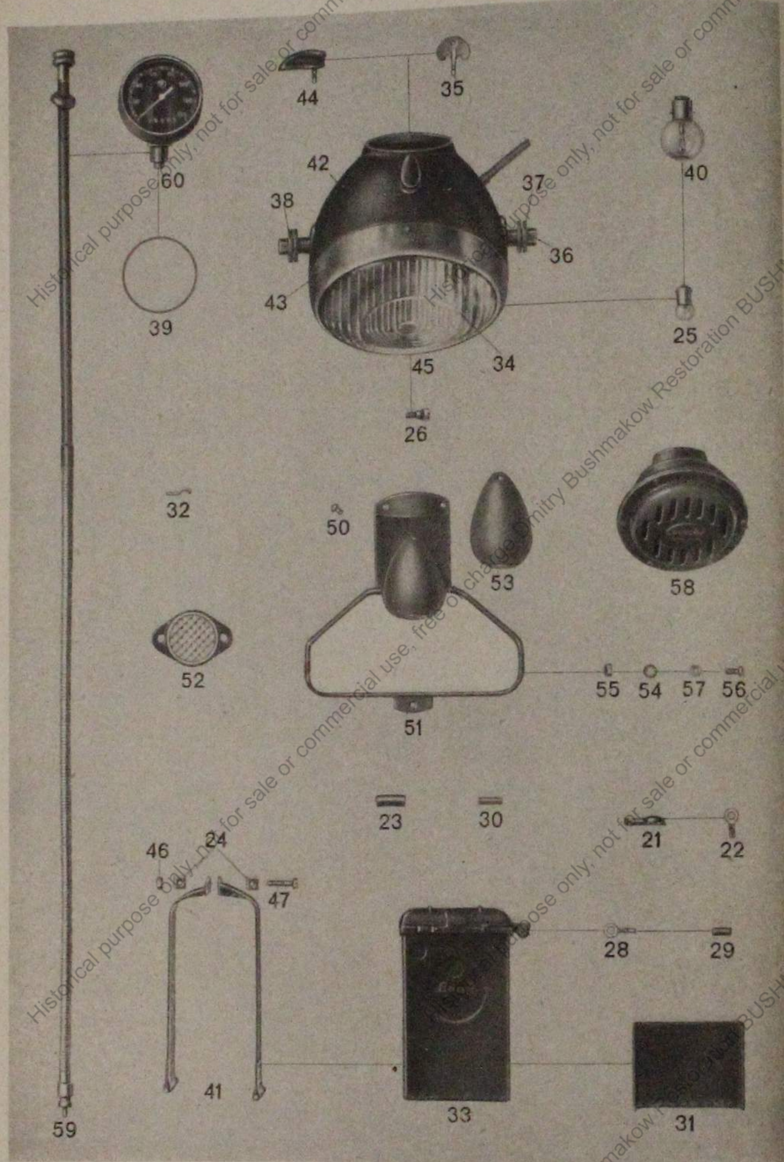
Tafel 27, Gruppe E: Zündlichtanlage
