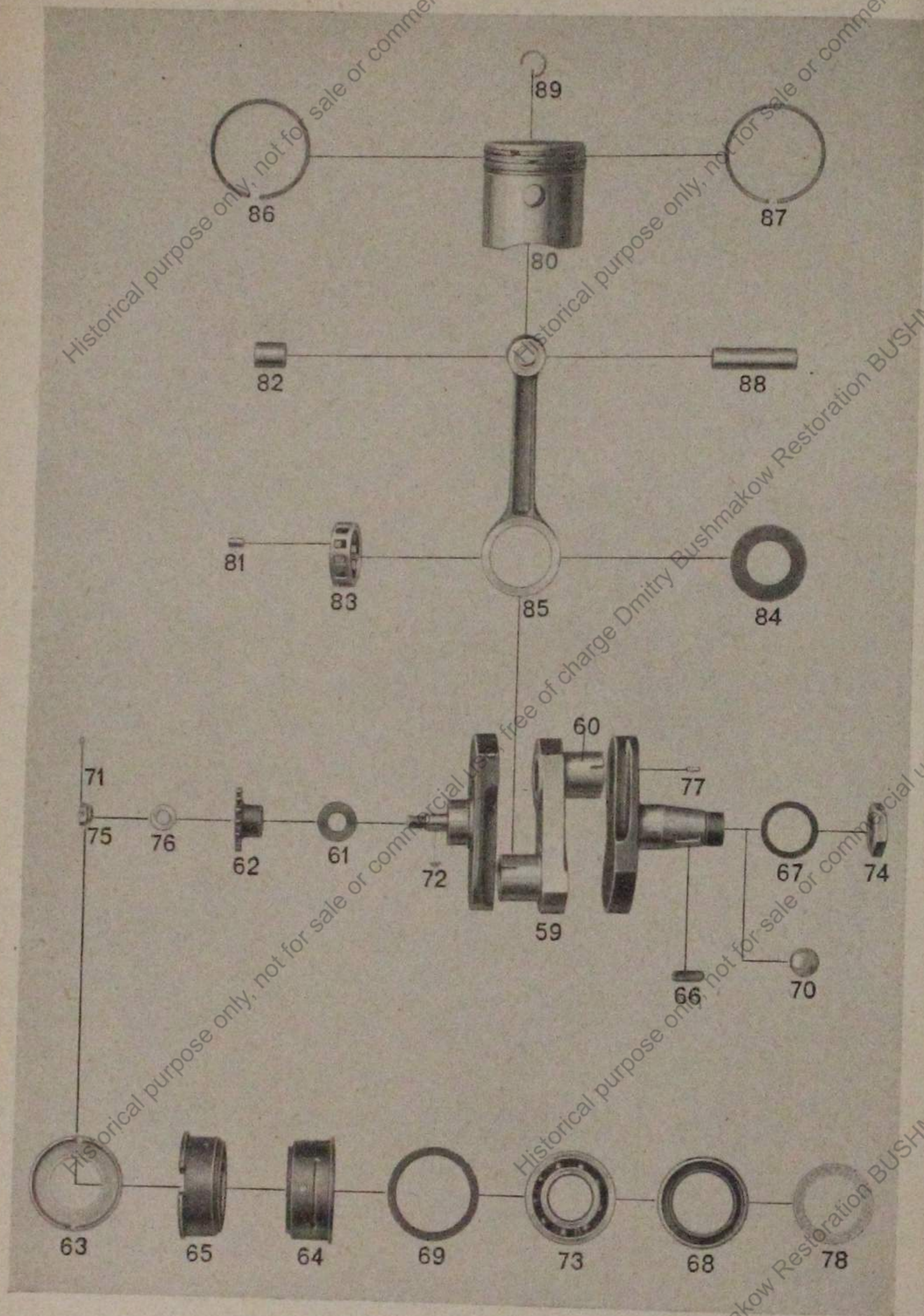
Tafel 4, Gruppe M: a) Motor, Triebwert
