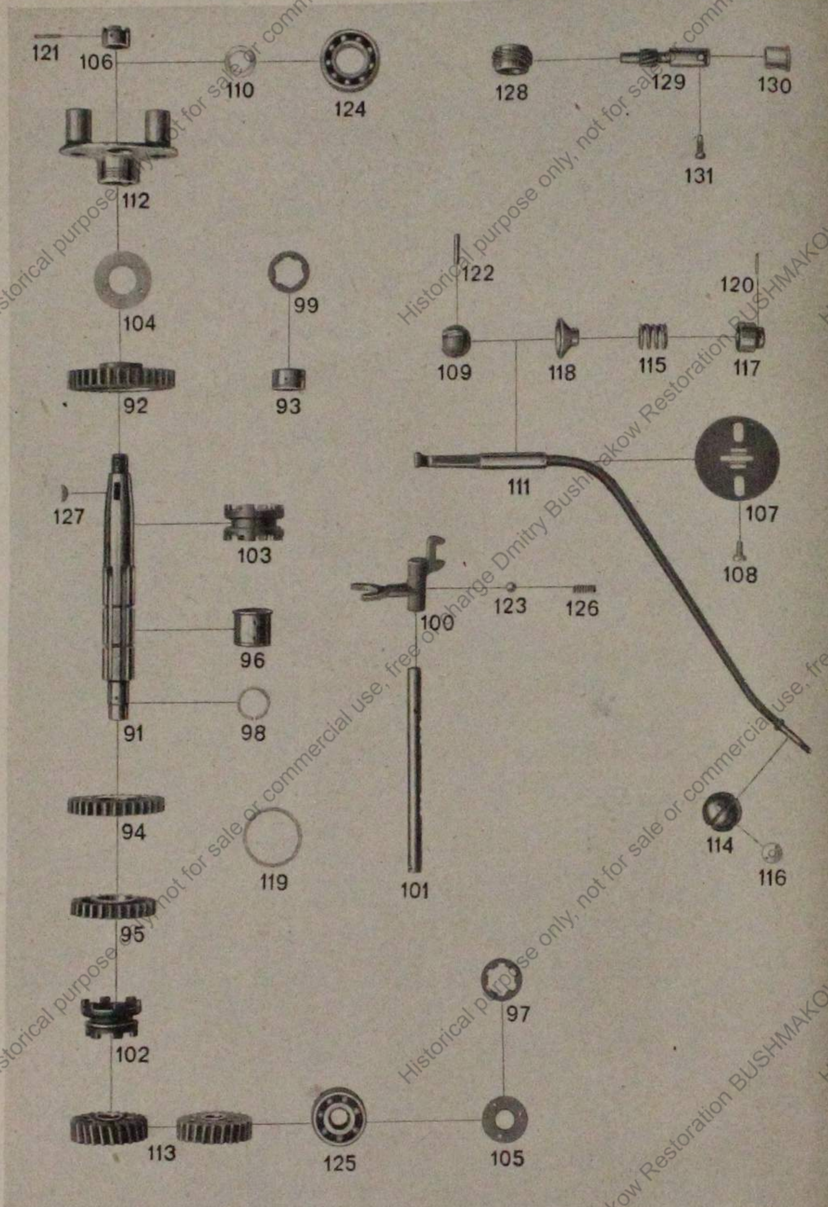
Tafel 11, Gruppe G: Wellen, Räder und Wegzählerantrieb
