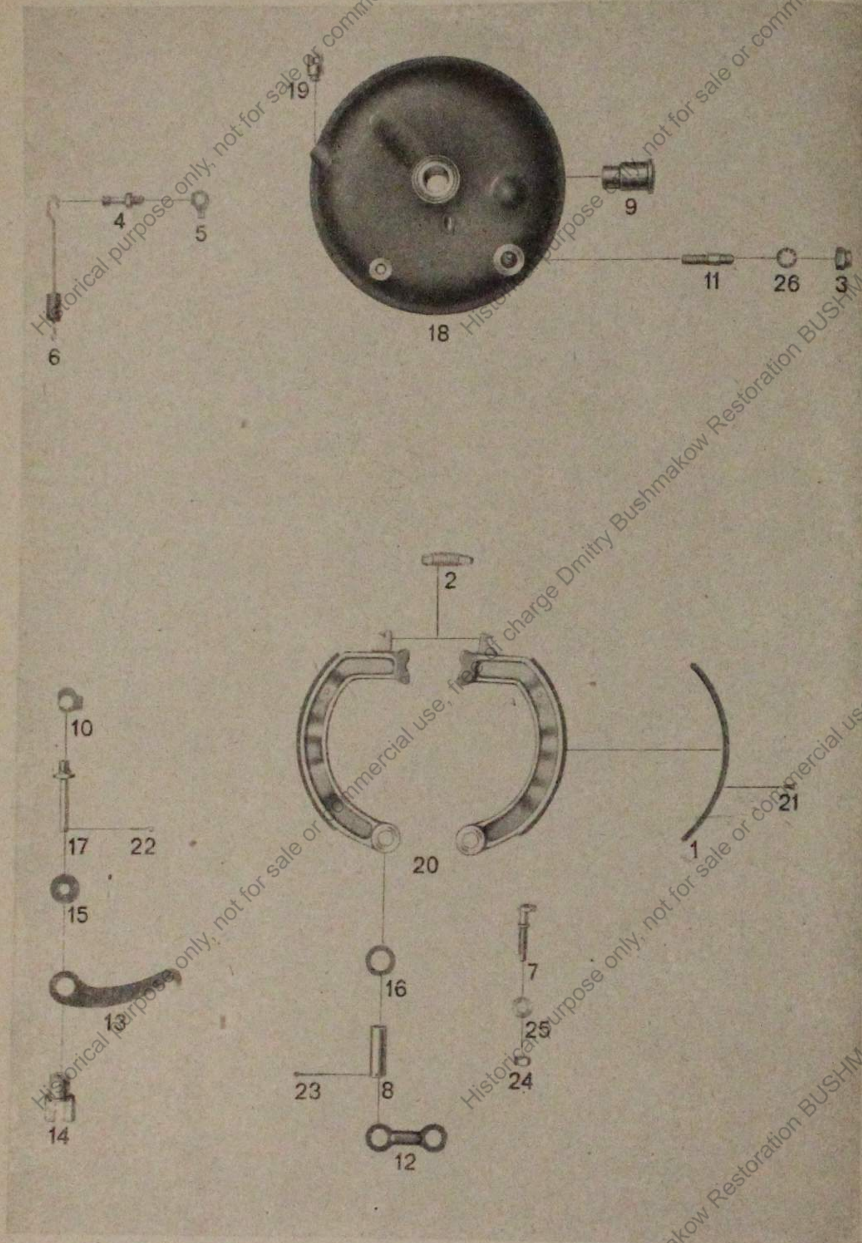
Tafel 22, Gruppe B: Bremsbetätigung Vorderrad
