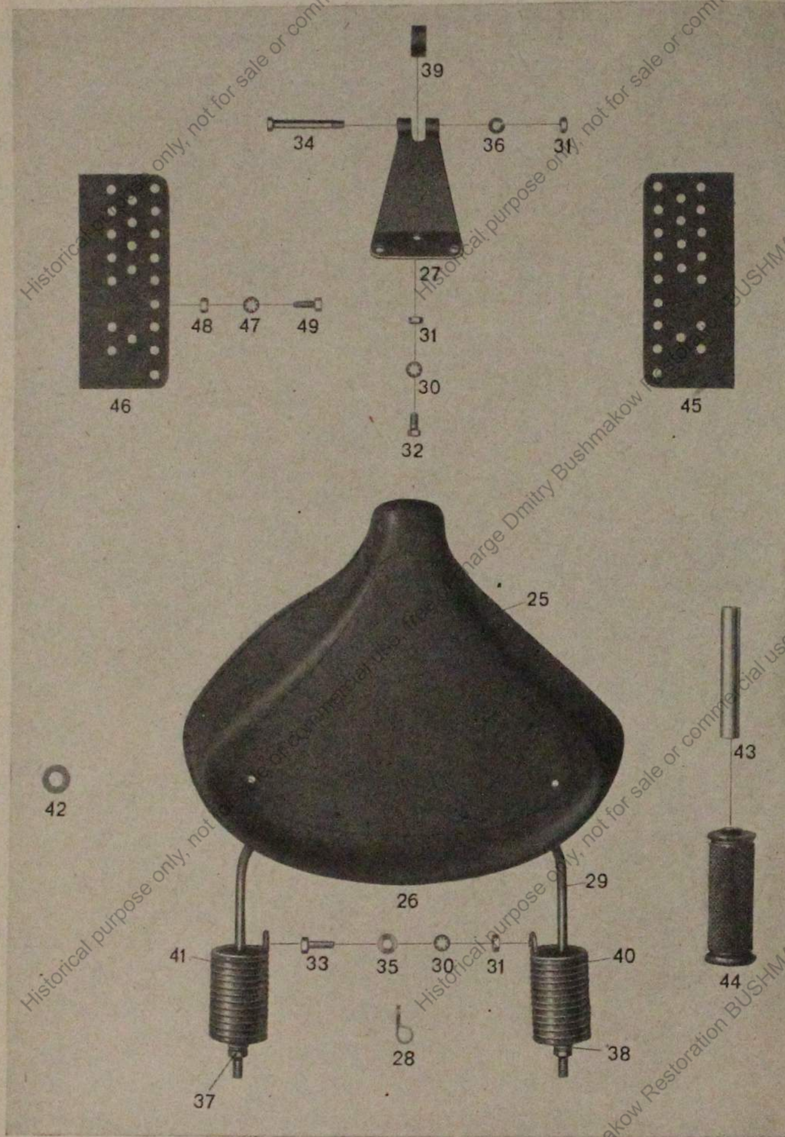
Tafel 13, Gruppe R: Sattel, Fußrasten
