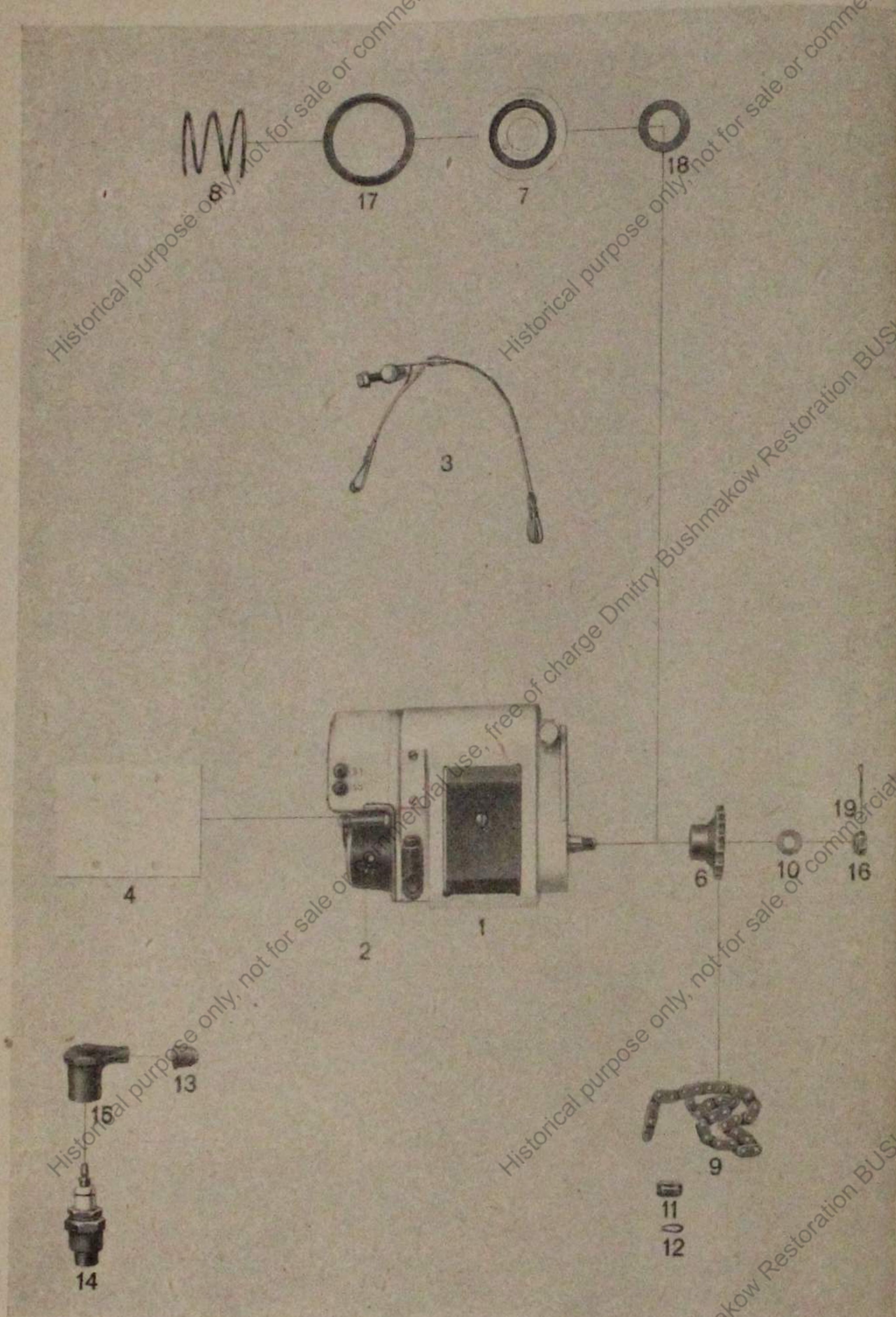
Tafel 26, Gruppe E: Zündung
