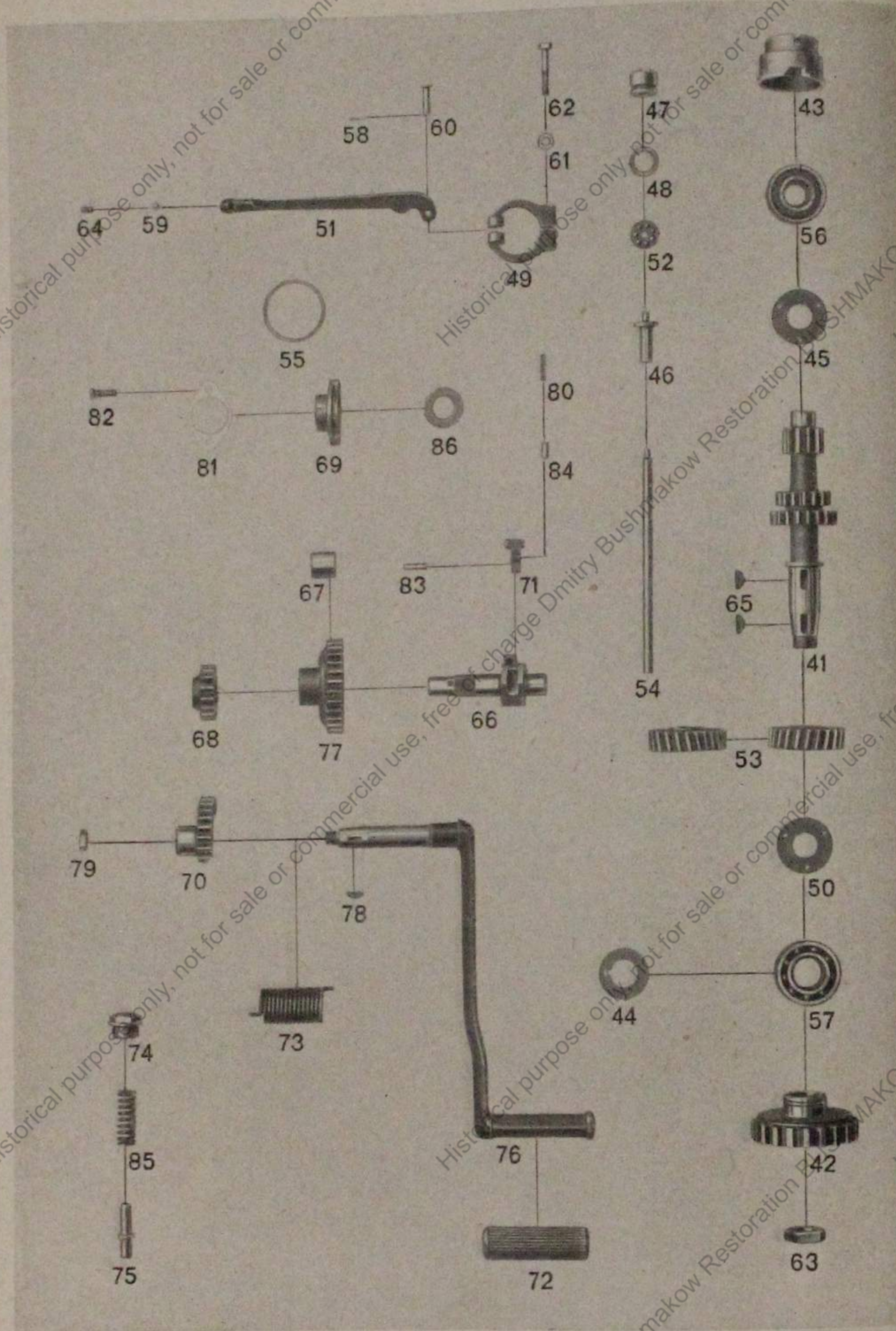
Tafel 10, Gruppe G: Wellen, Zahnräder und Kiststarter
