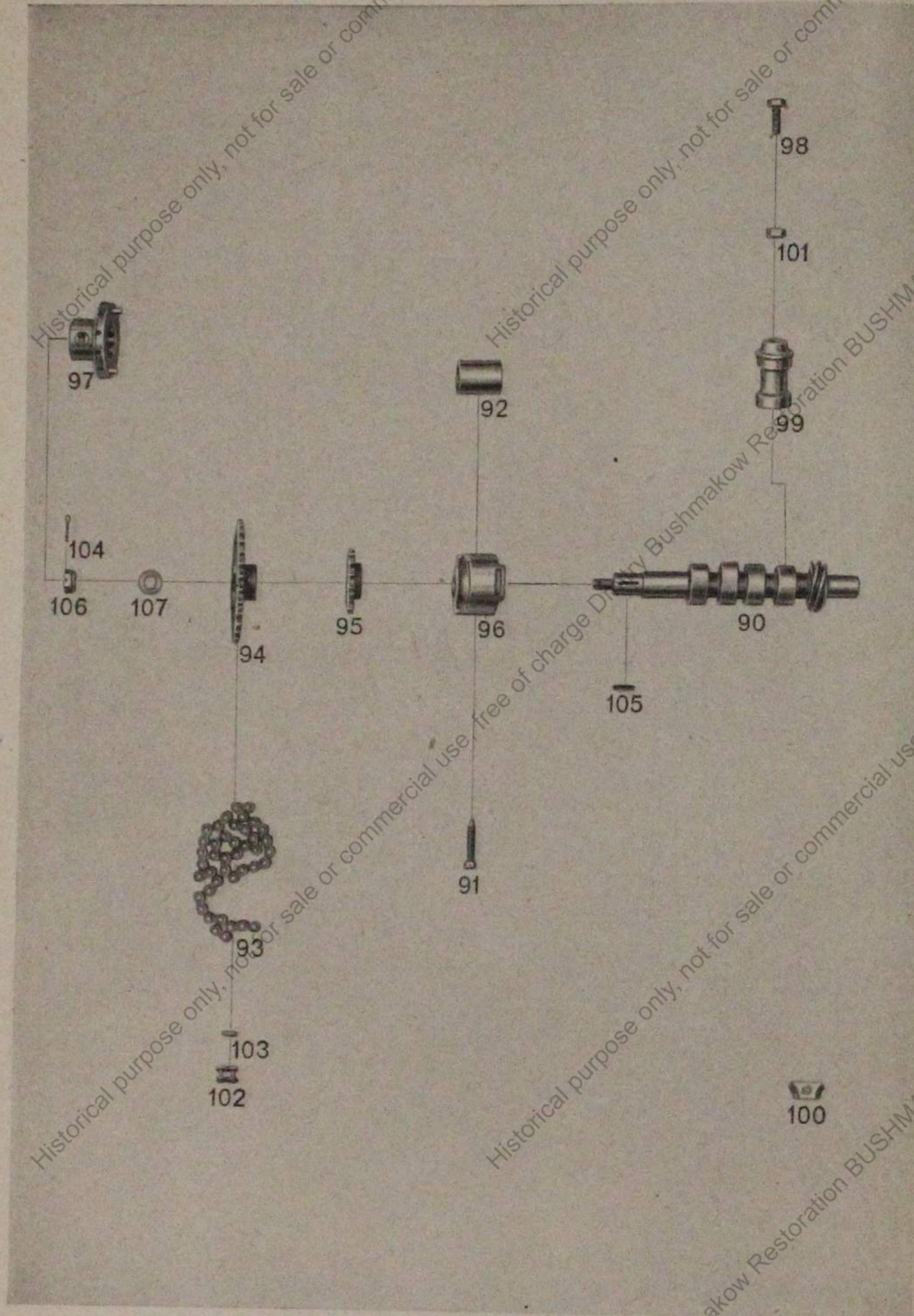
Tafel 5, Gruppe M: a) Motor, Ventilsteuerung
