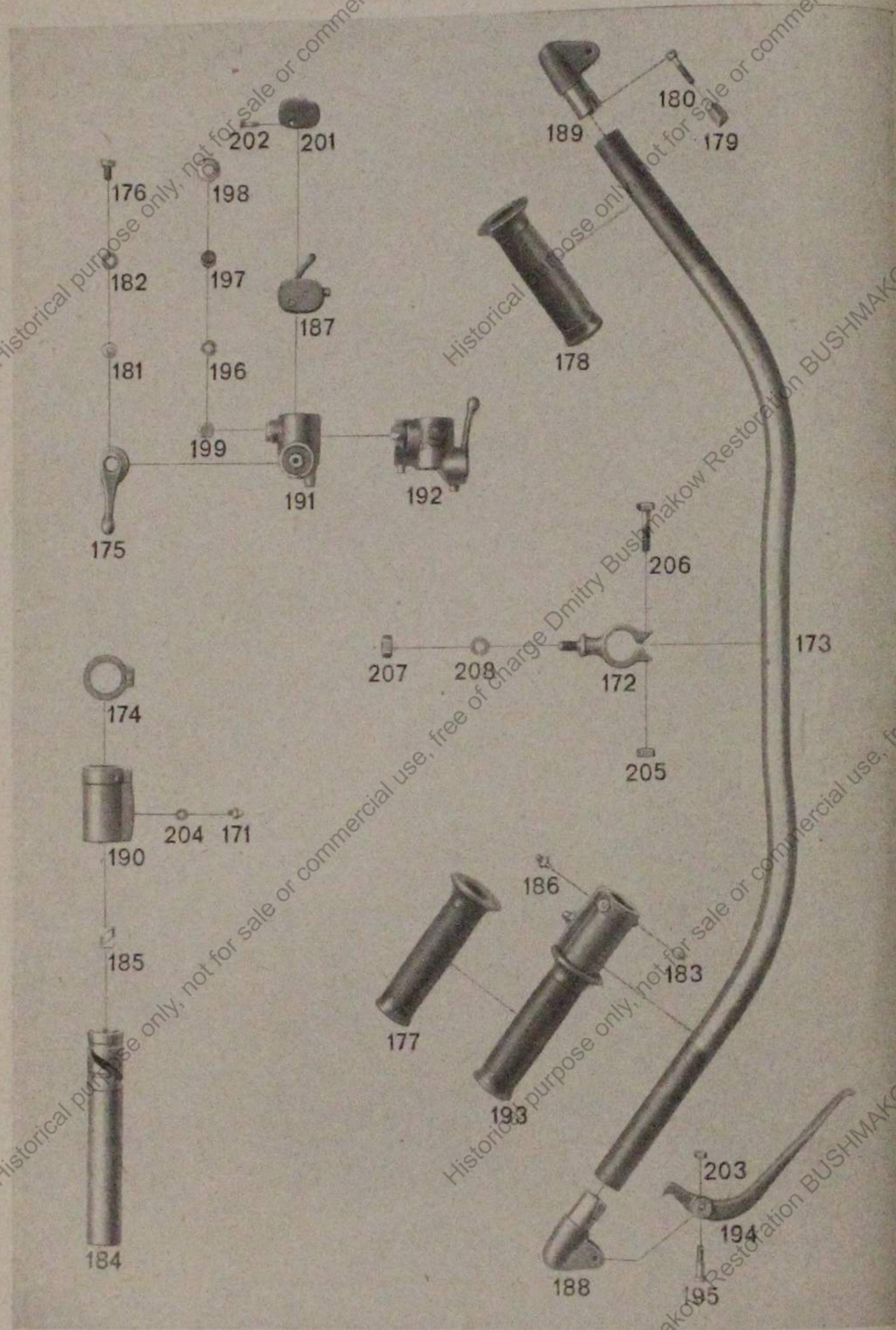
Tafel 20, Gruppe R: Lenker mit Betätigungen
