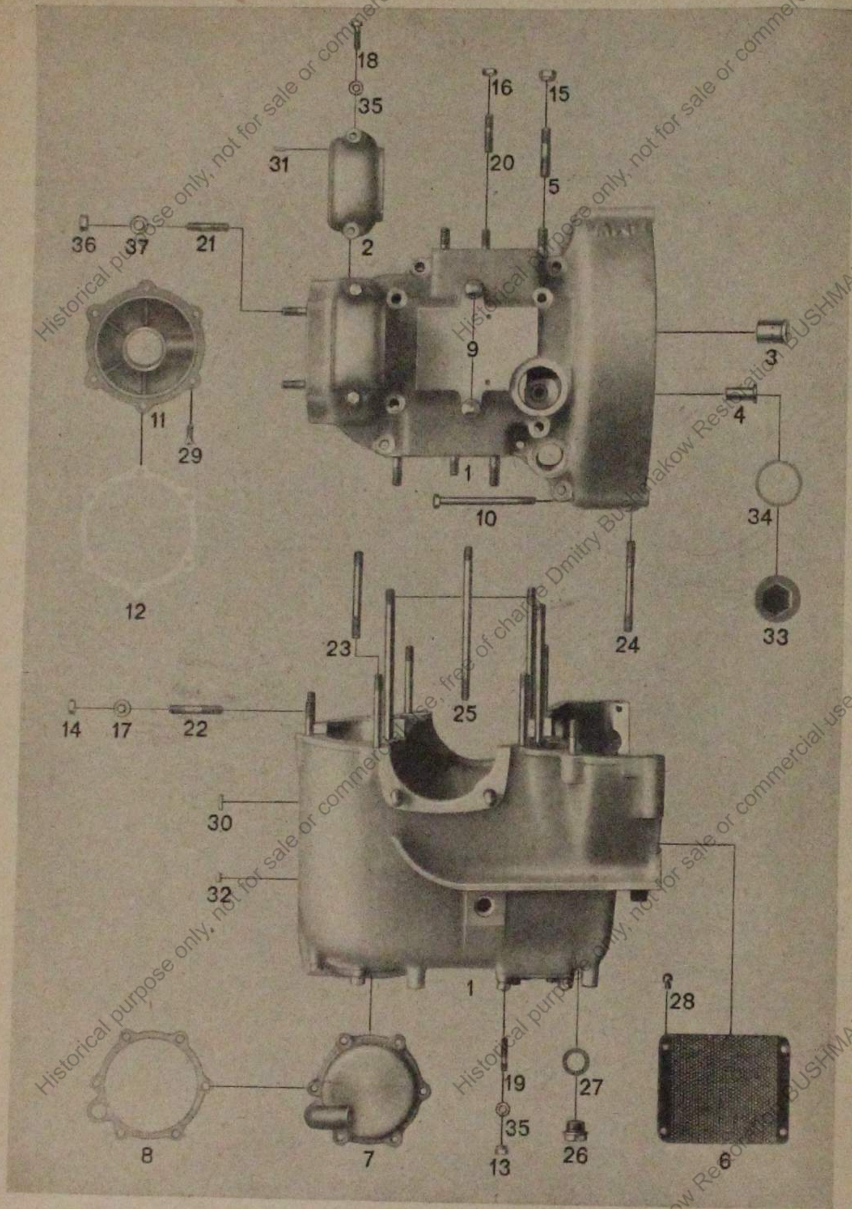
Tafel 2, Gruppe M: a) Motor, Motorgehäuse
