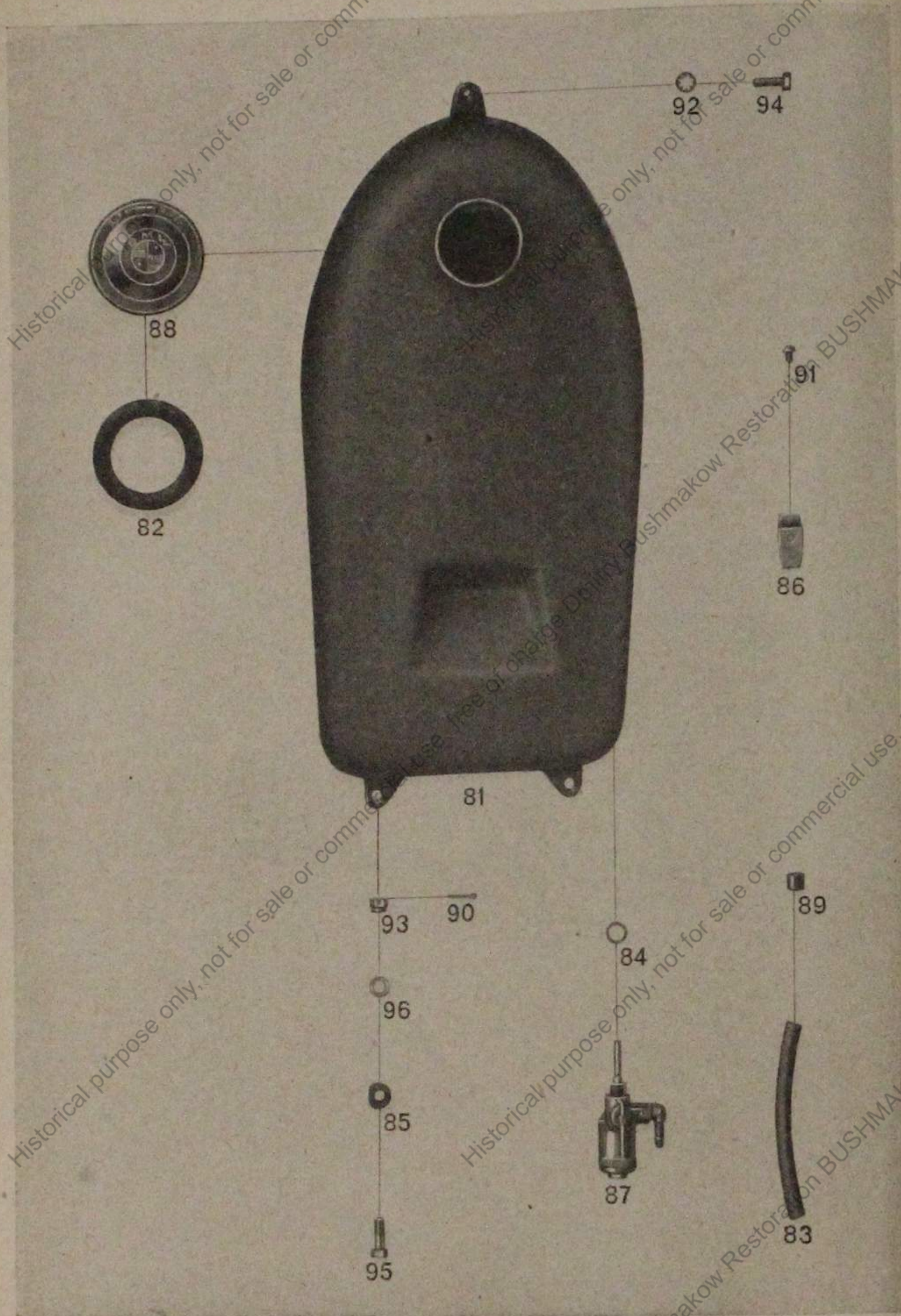
Tafel 16, Gruppe R: Kraftstoffbehälter mit Leitung
