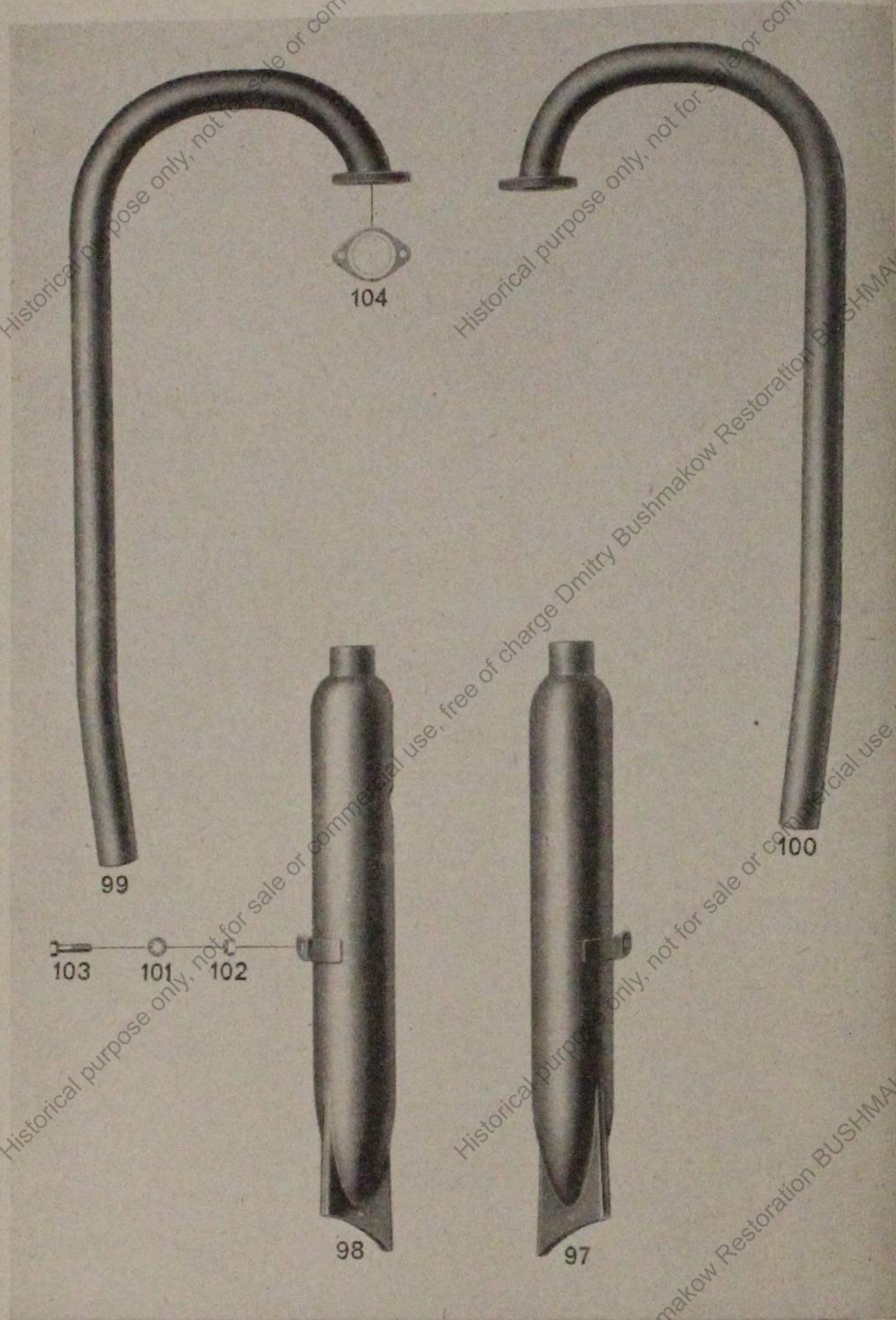
Tafel 17, Gruppe R: Auspufftopf und Leitung
