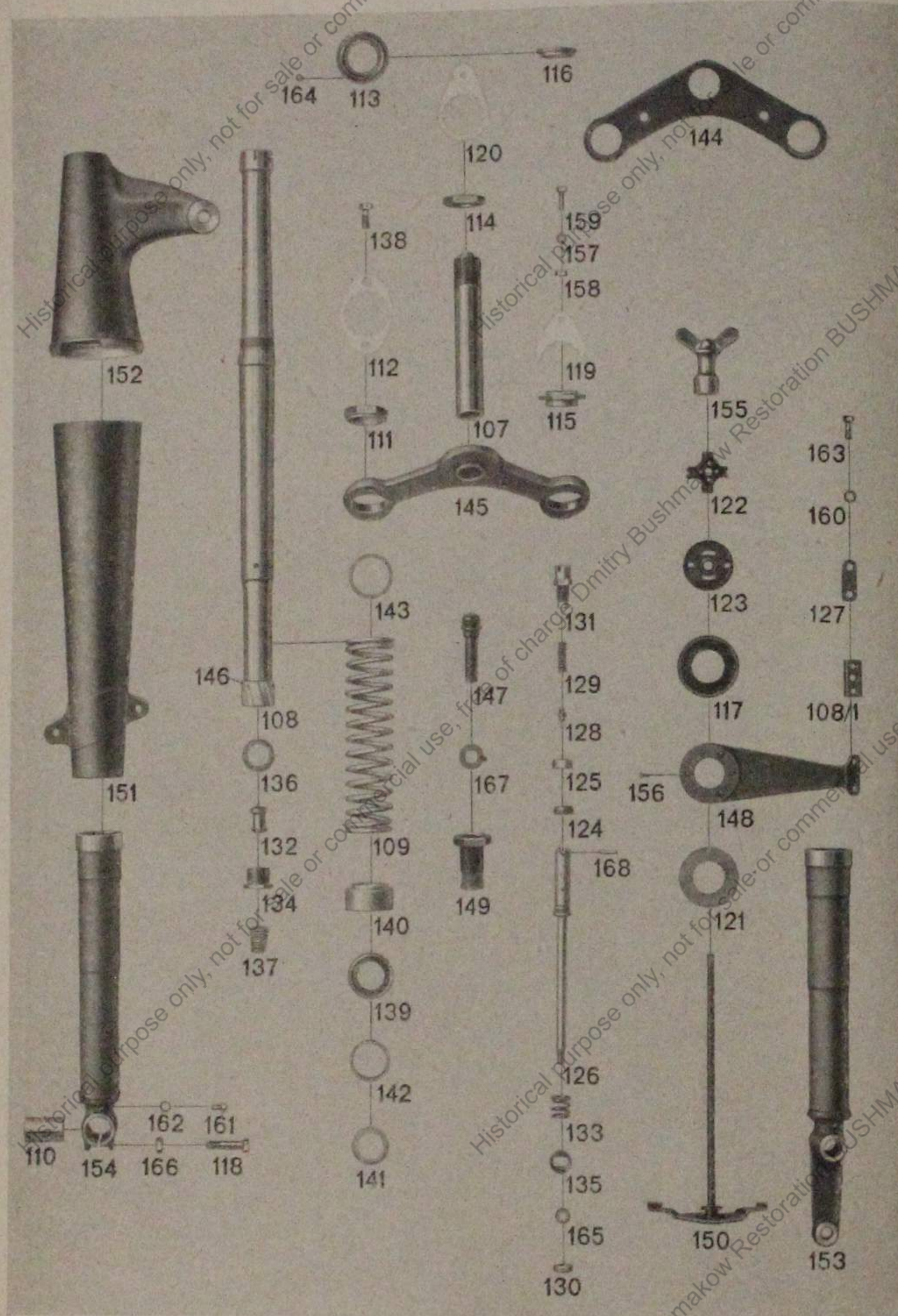
Tafel 19, Gruppe R: Federgabel
