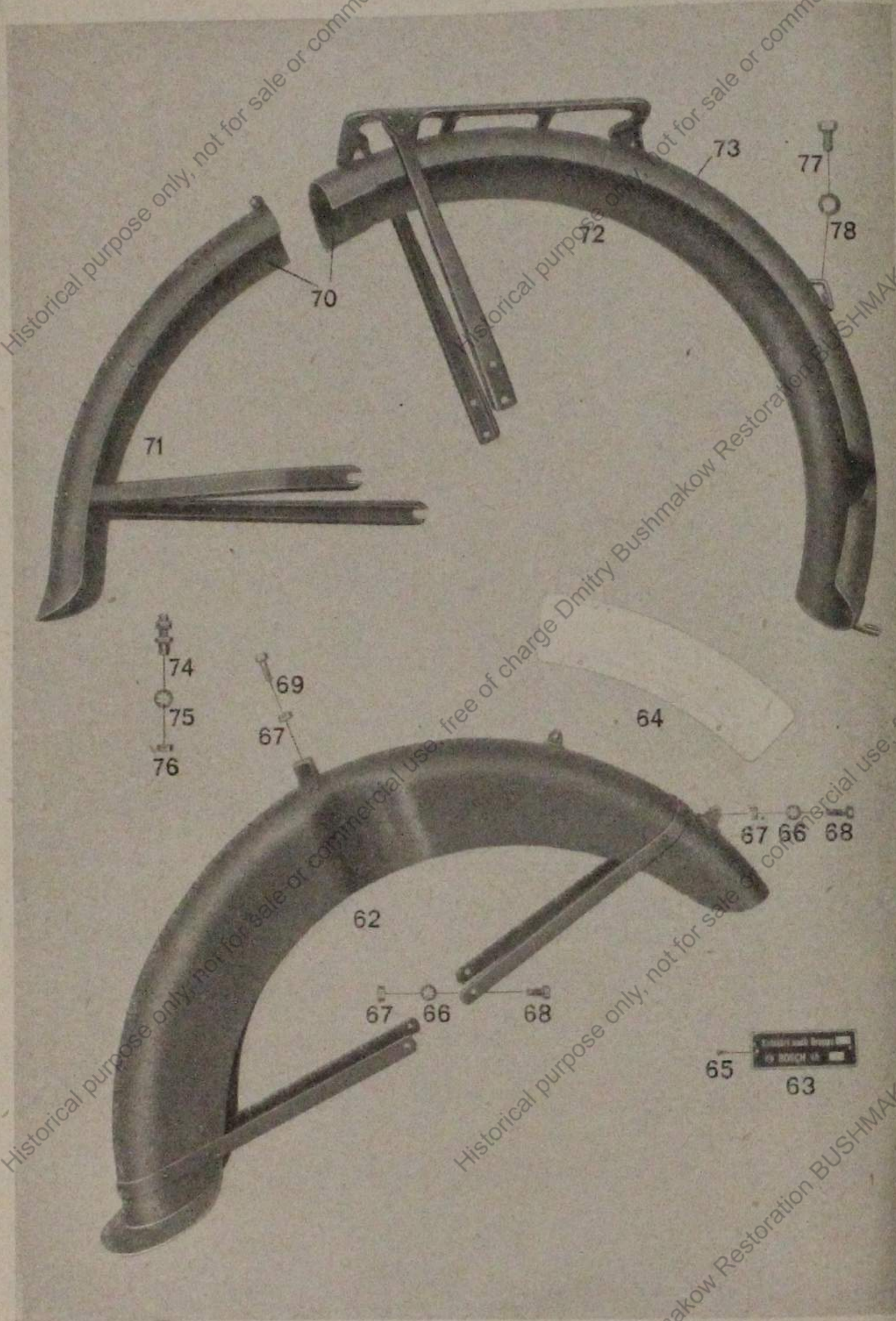
Tafel 15, Gruppe R: Kotflügel
