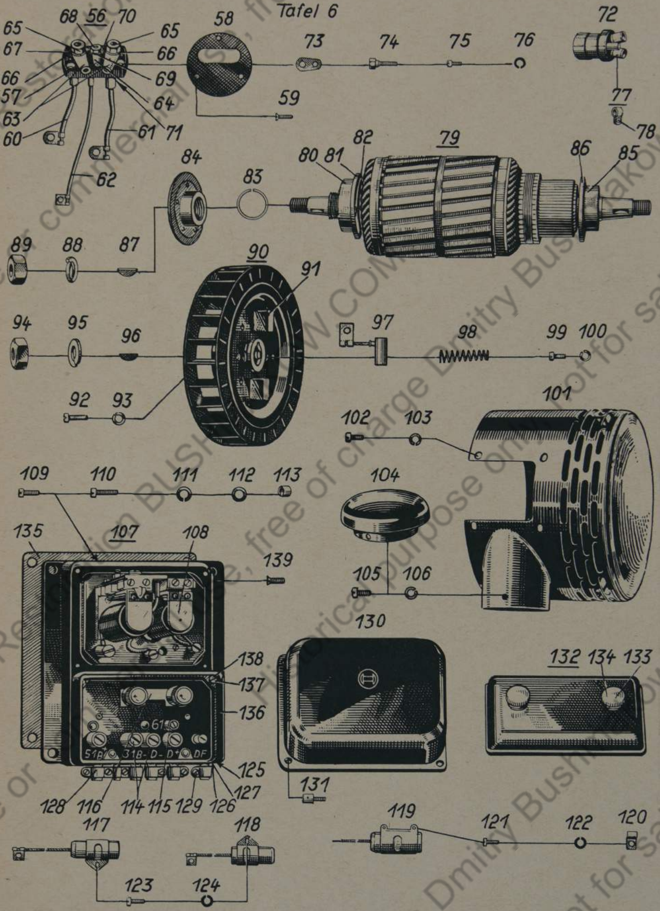
Gruppe: Lichtmaschine GTL 600/12/1200 RS 41
