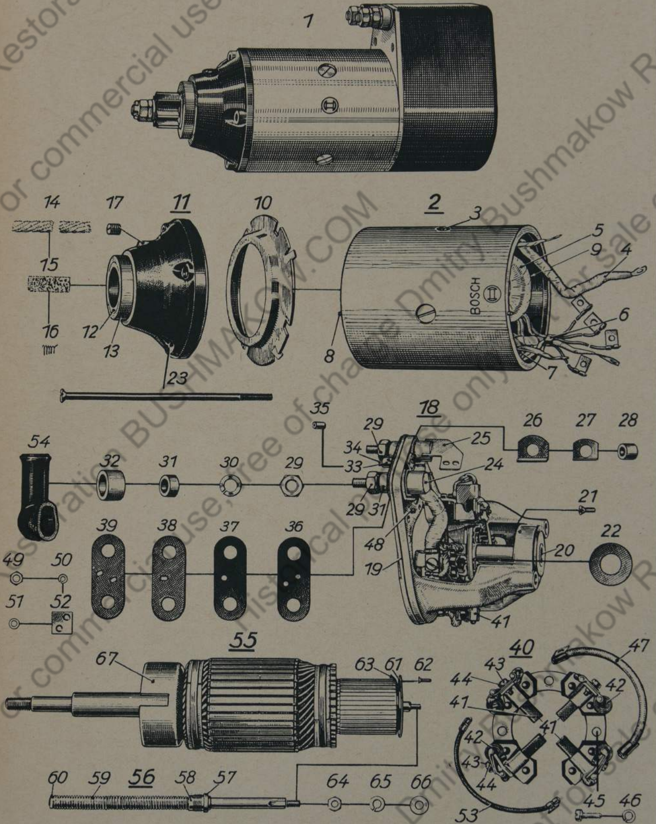
Gruppe: Anlasser BNG 4/24 AR 9 Z 11
