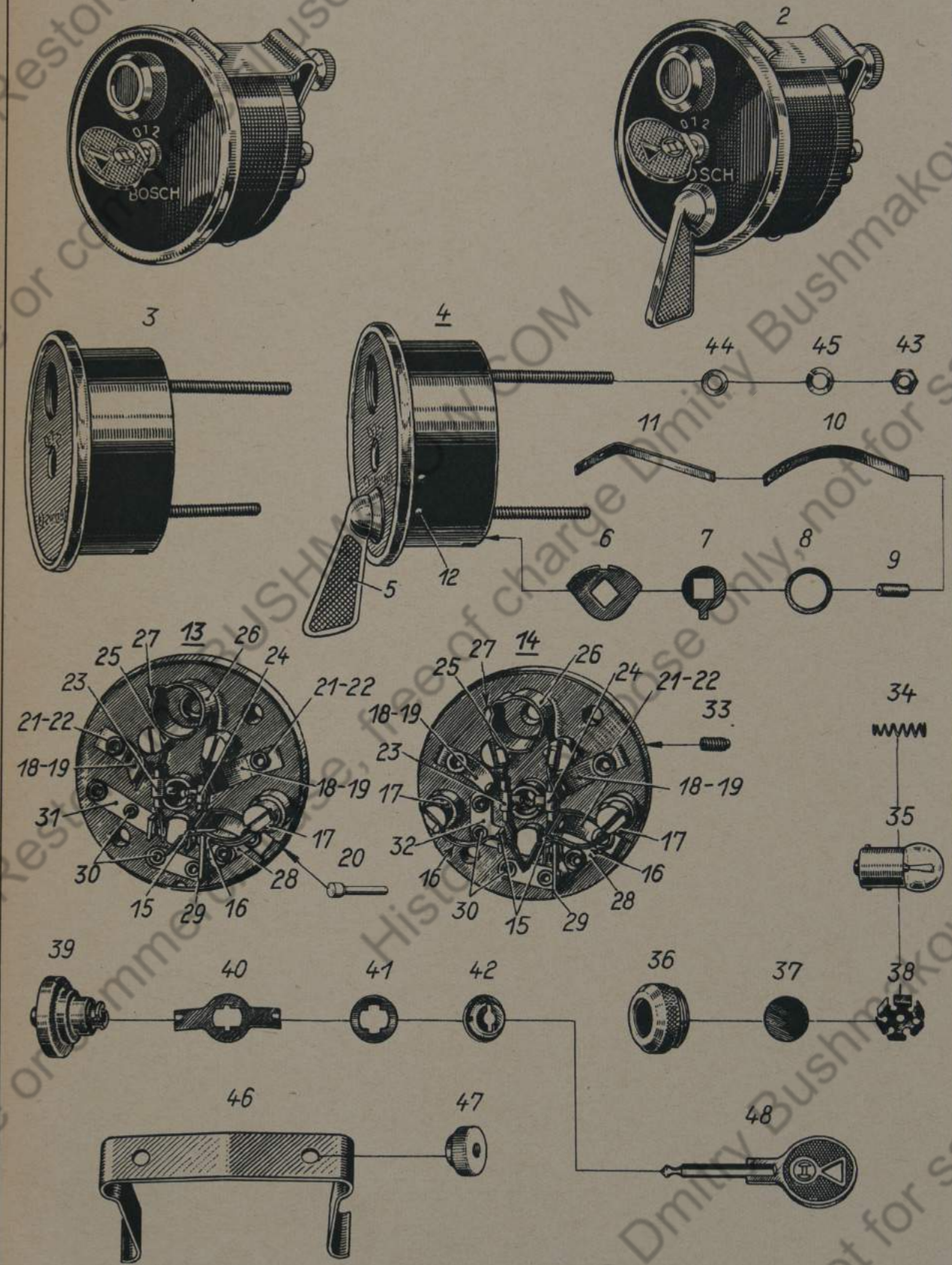
Gruppe: Schaltkasten HA 12 S13 und S 27
