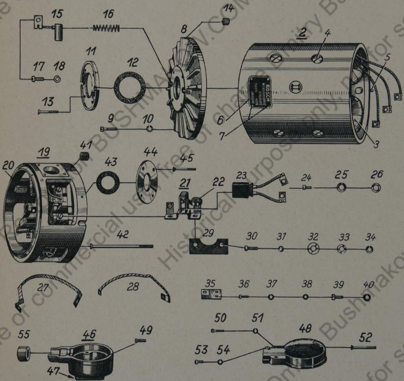
Gruppe: Lichtmaschine GTL 600/12/1200 RS 41
