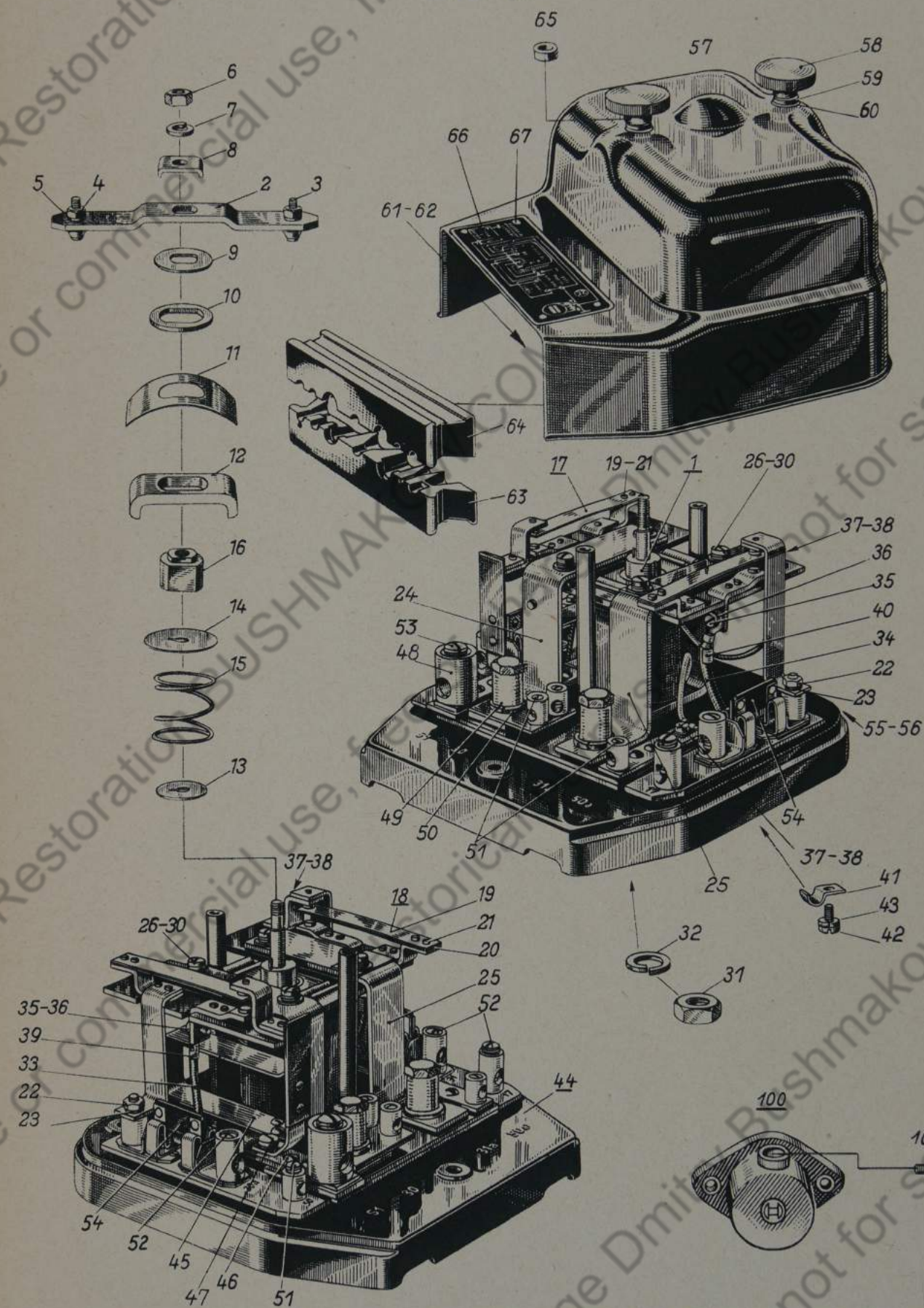
Gruppe: Batterieschalter SSM 108/1Z u. 4Z, Steckdose RS 155/3
