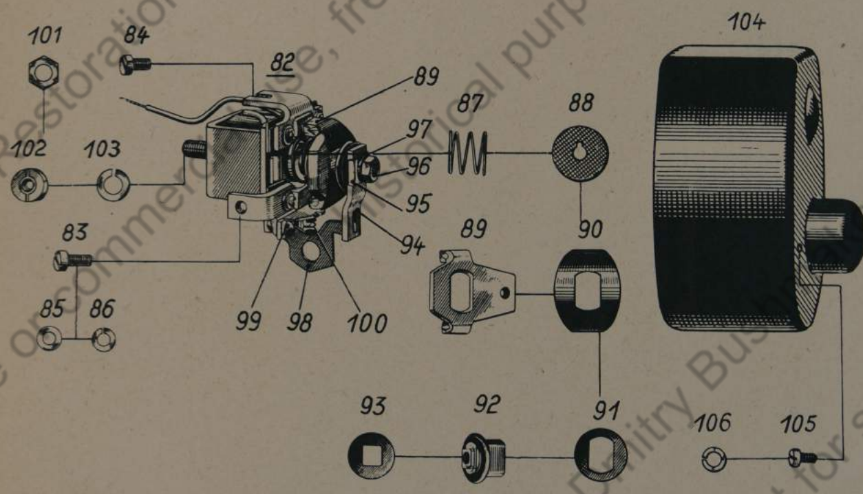
Gruppe: Anlasser BJH 14/12R3
