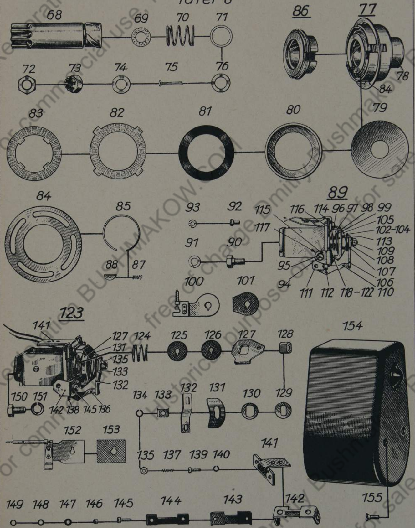
Gruppe: Anlasser BN6 4/24 AR9 Z 11
