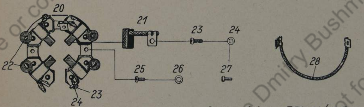
Gruppe: Anlasser BJH 14/12R3
