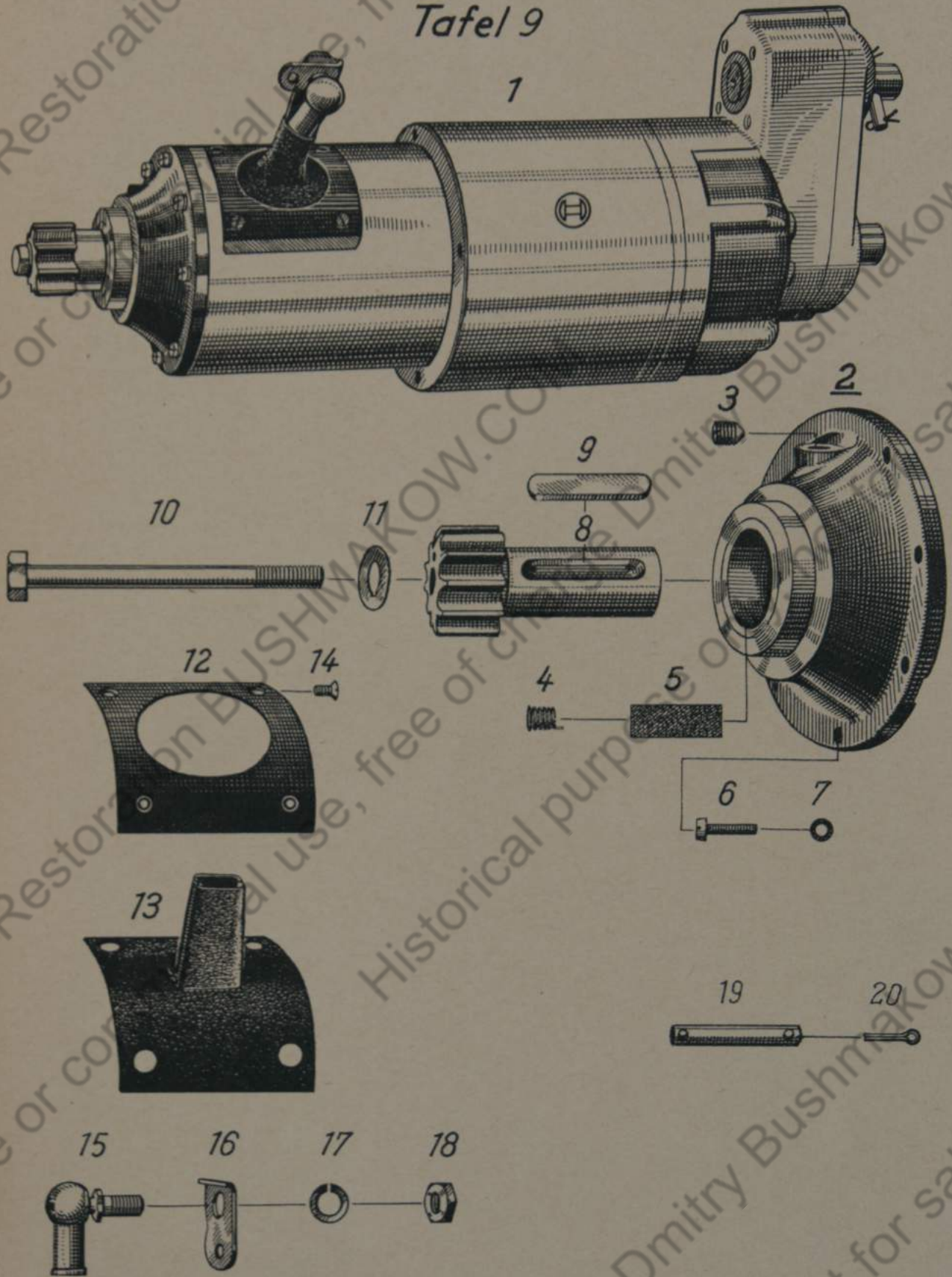
Gruppe: Schwungkraftanlasser AL/ZMA
