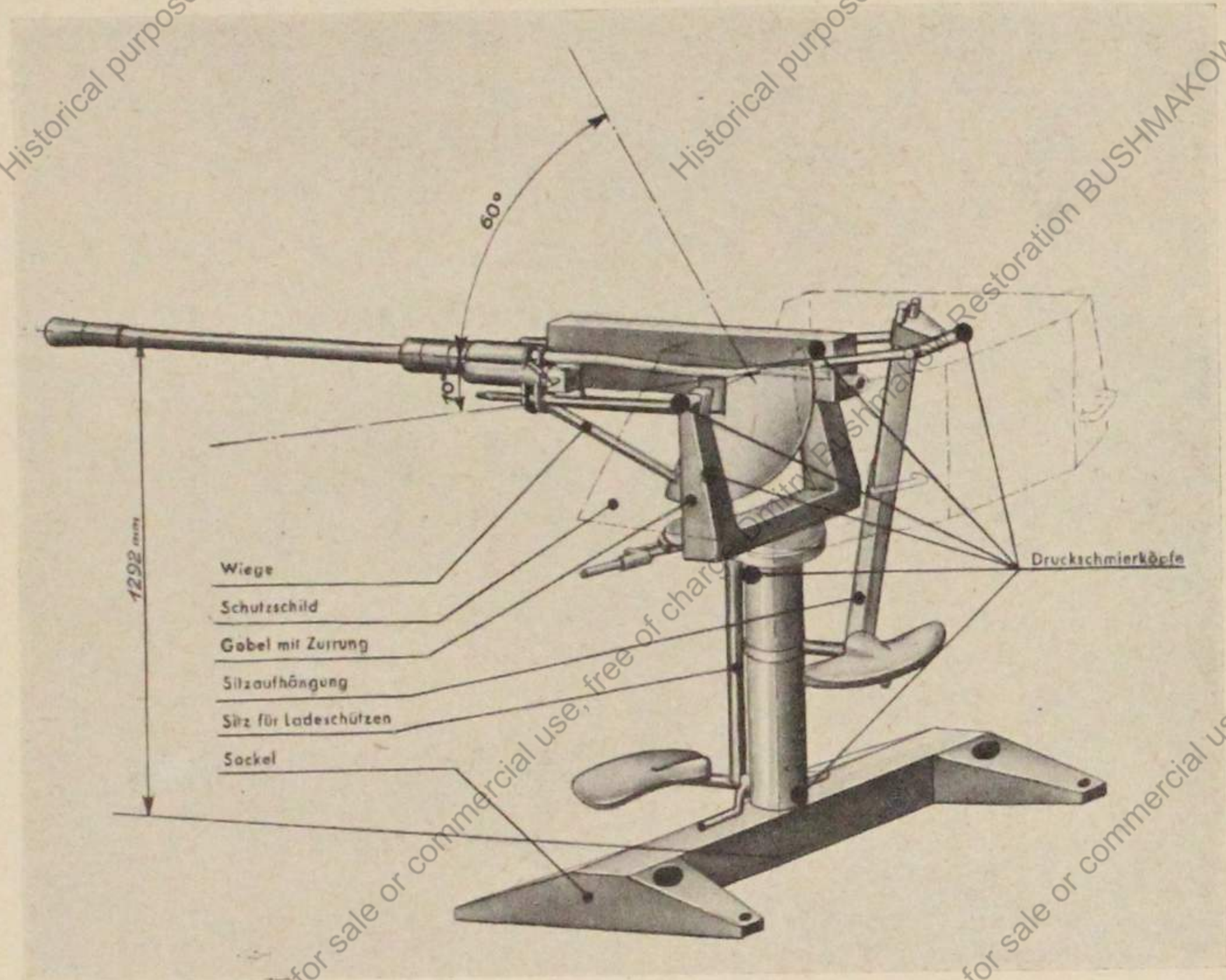
Bild 1 2 cm Schwebelafette 38 mit Schmierstellen
