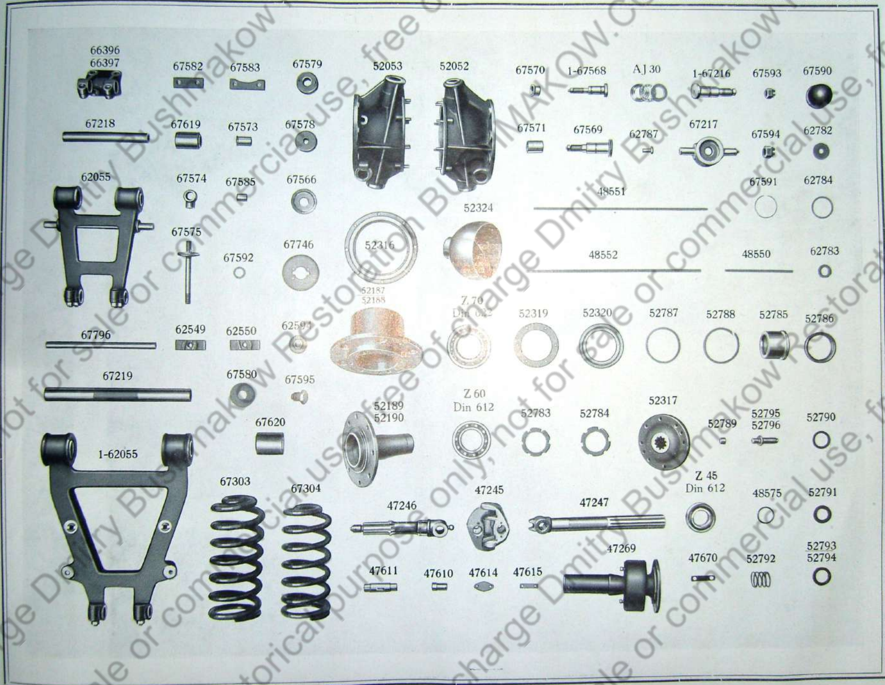
TAFEL 8: EINZELRADAUFHÄNGUNG
