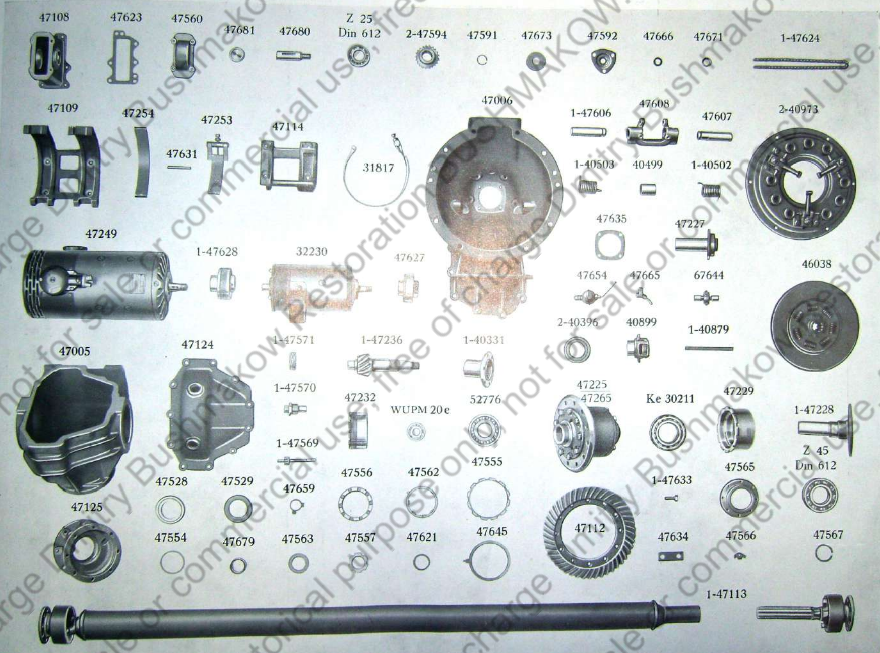
TAFEL 5: GETRIEBE UND KUPPLUNG
