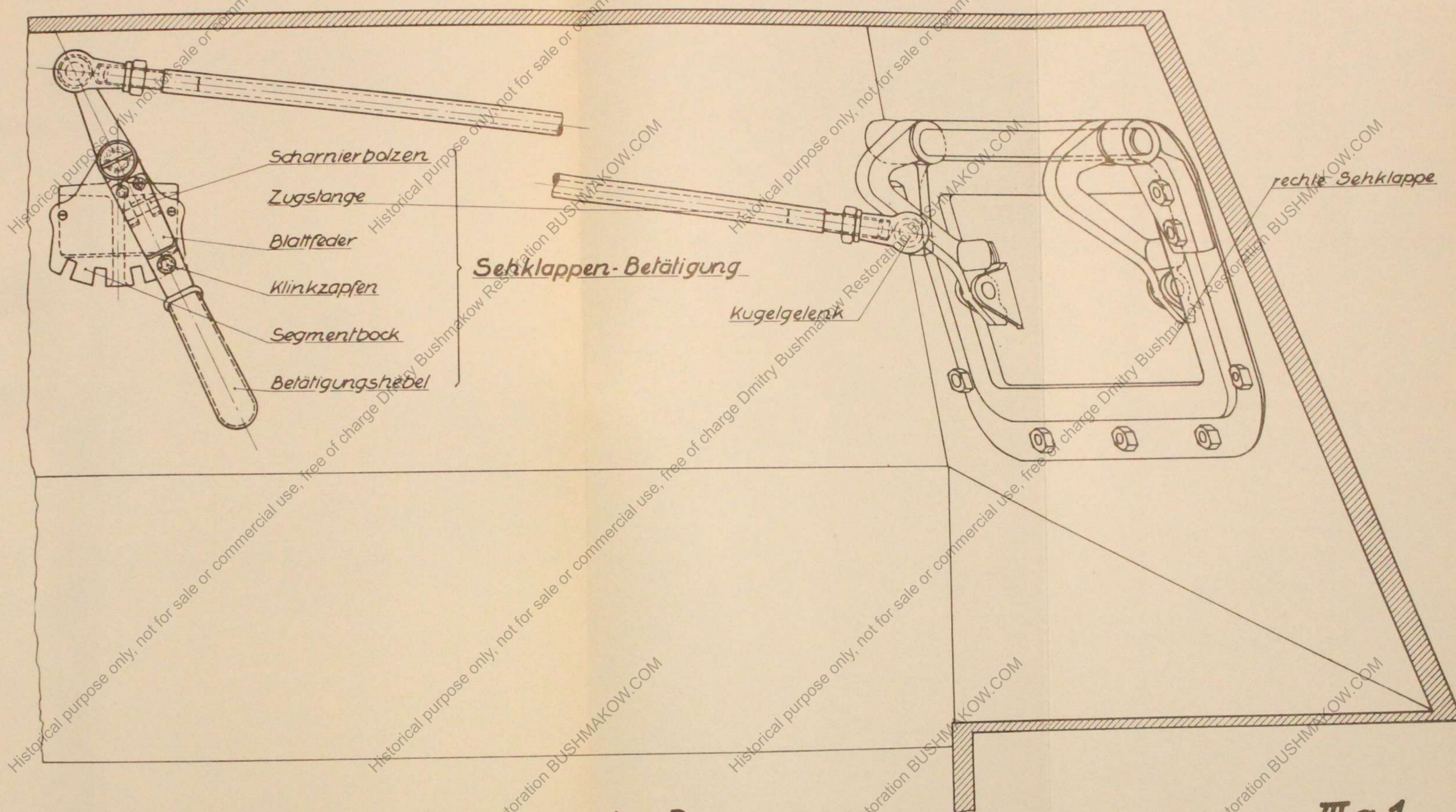
Rechte Sehklappe im Bugpanzer.
