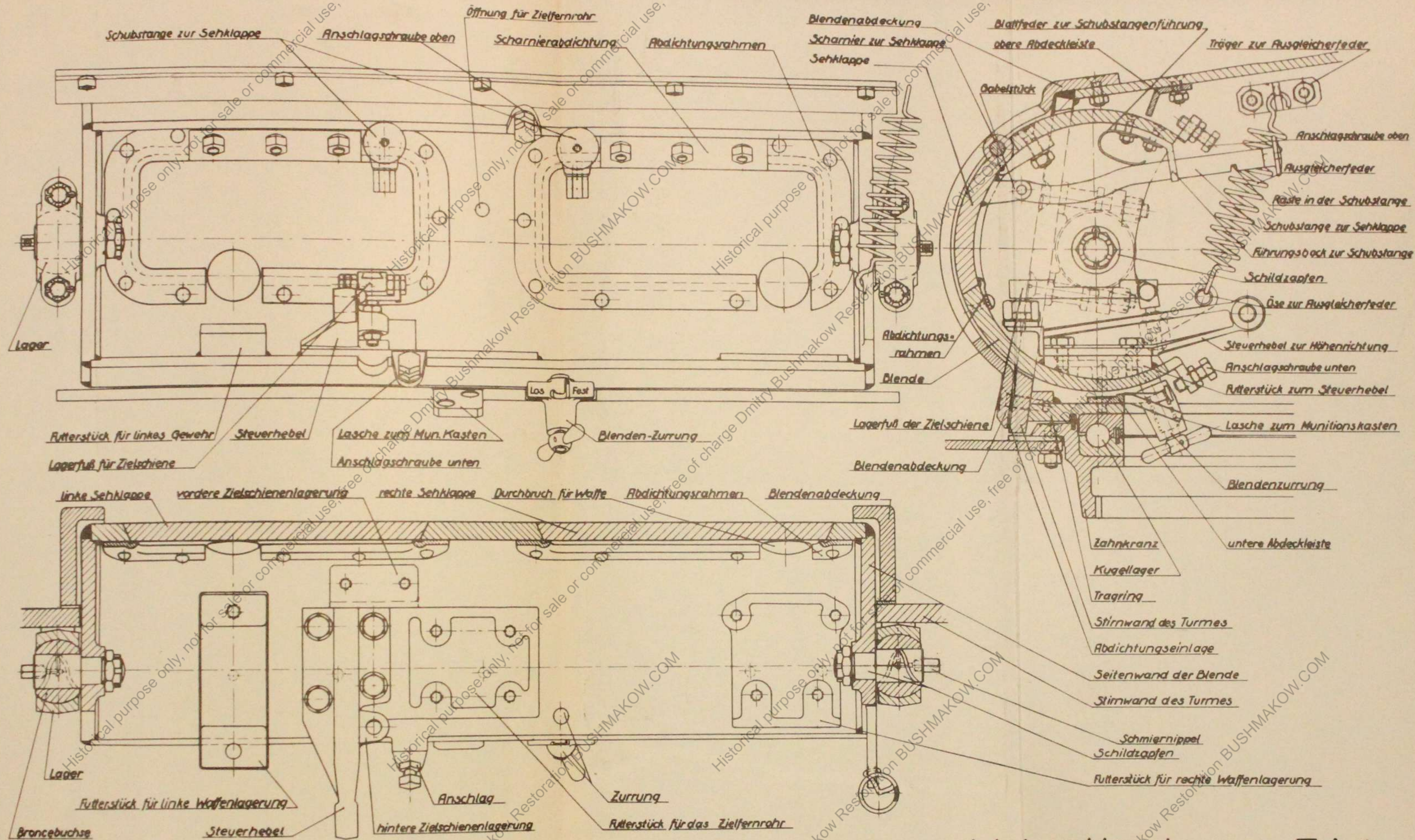
Walzenblende
