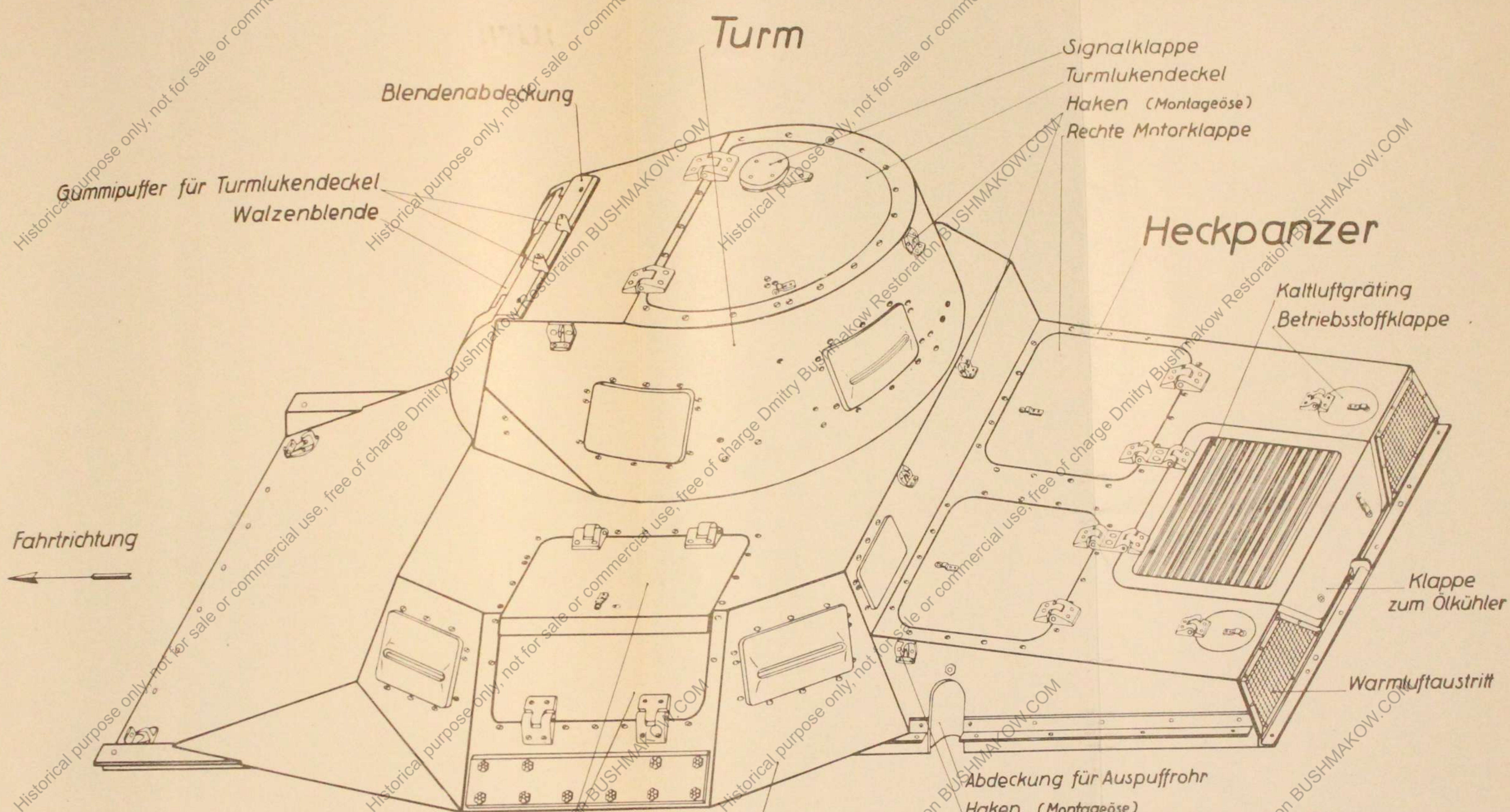
Der Aufbau zum Pz. -Kampfwagen II.a. (Bild 1)
