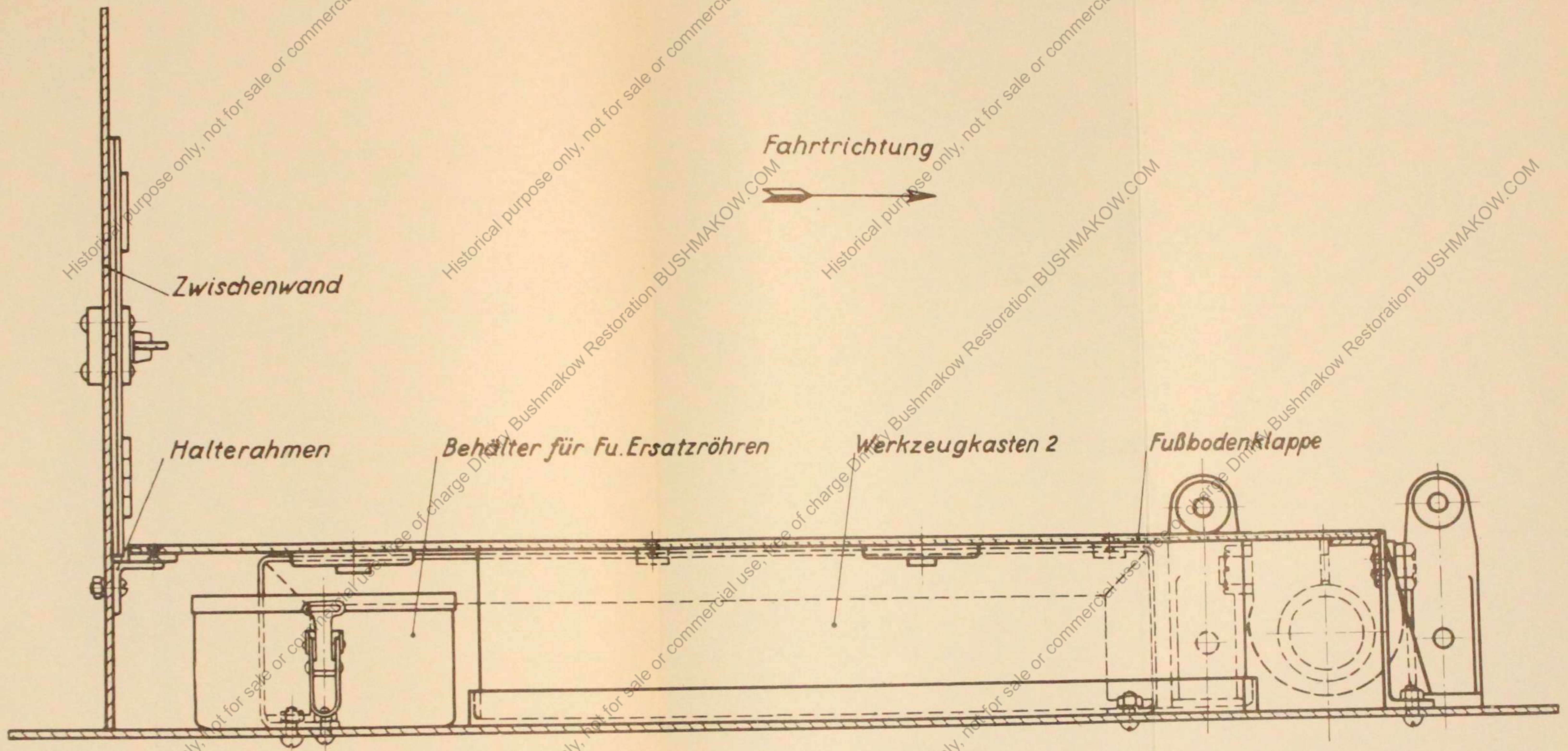
Linker Fußboden Schnitt E - F
