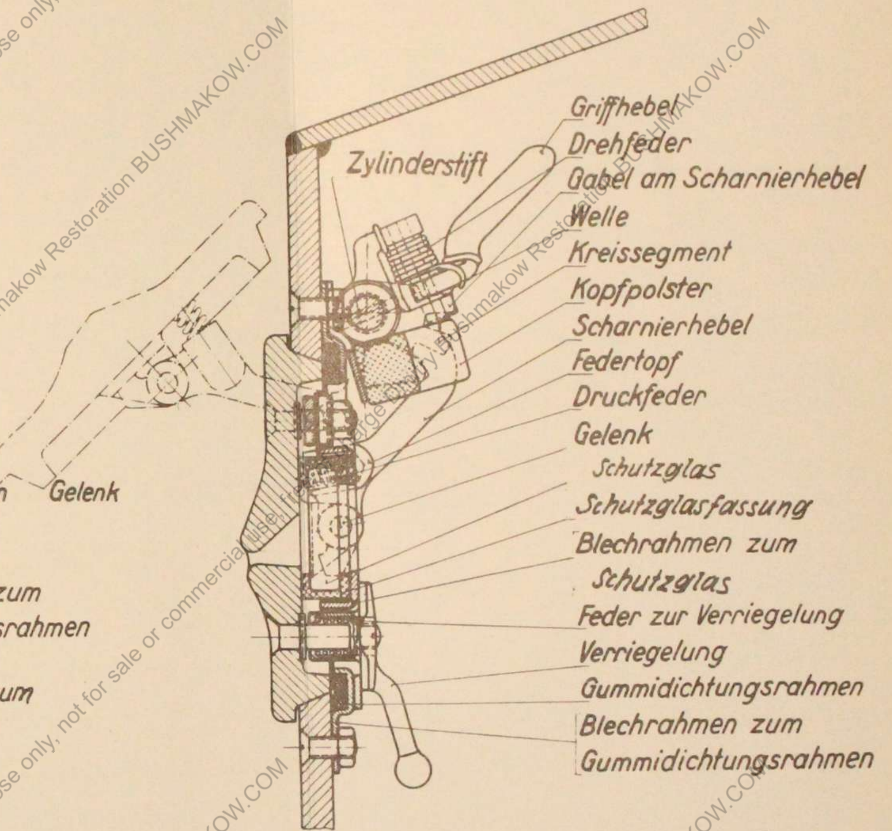
III. a.1 (Bild 1)
