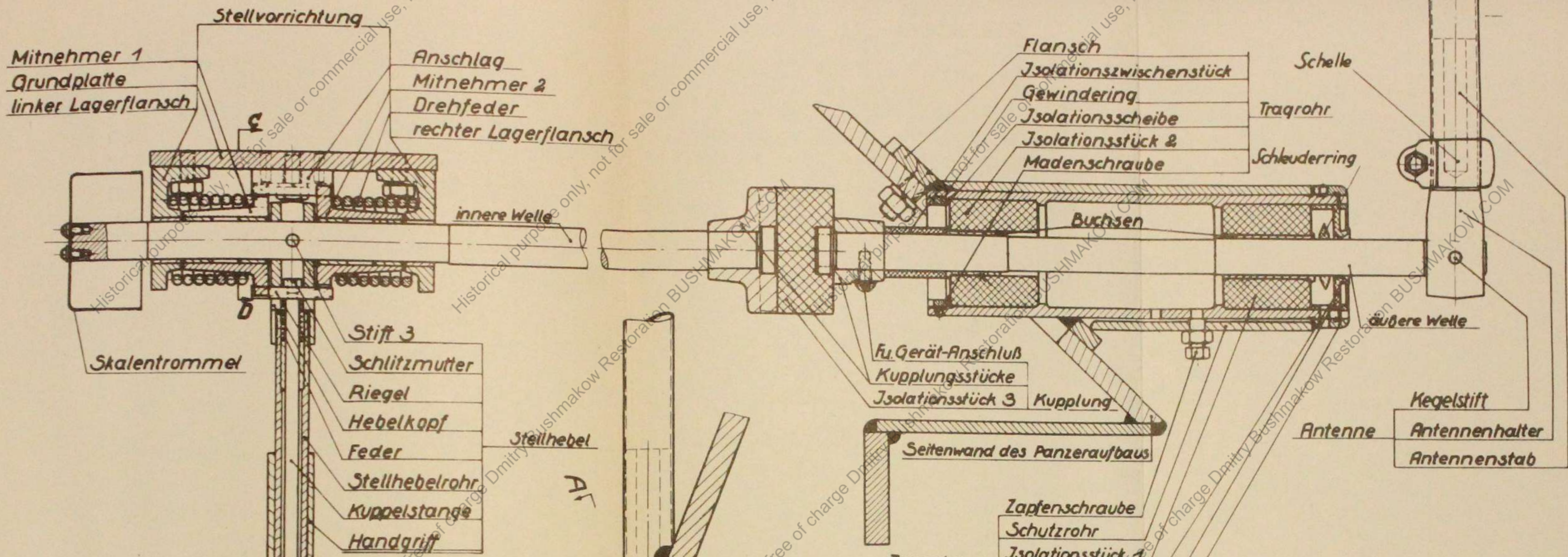
Schnitt A-B
