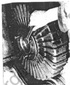
Bremstrommel mit 3 Abdrückschrauben 14×90 (SW 22) abdrücken.
