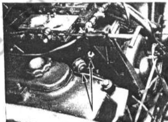
Einstellung der Düsen am vorderen Vergaser.
