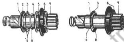
Zusammenbau des Ritzelschaftes
