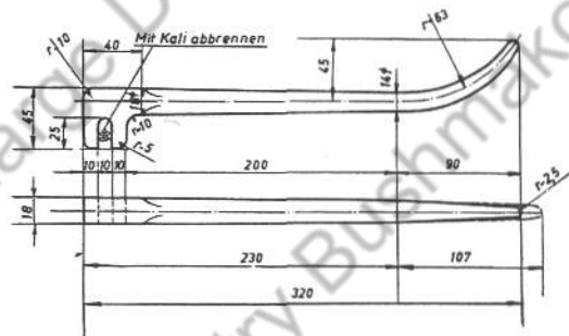
Rechtwerkzeug für Schalthebel Zeichn. Nr. W 212/2.
