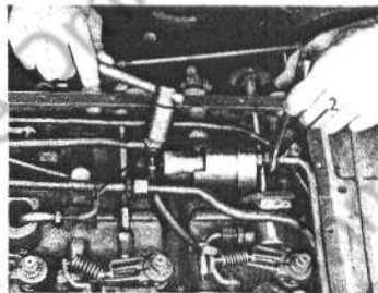
Doppelhohlschraube (1) am Akkumulator mit Steckschlüssel SW 19 abnehmen.
