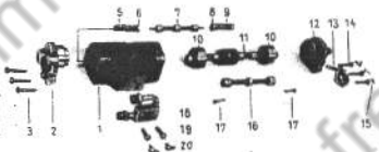
Schaltzylinder III zerlegt und gereinigt
