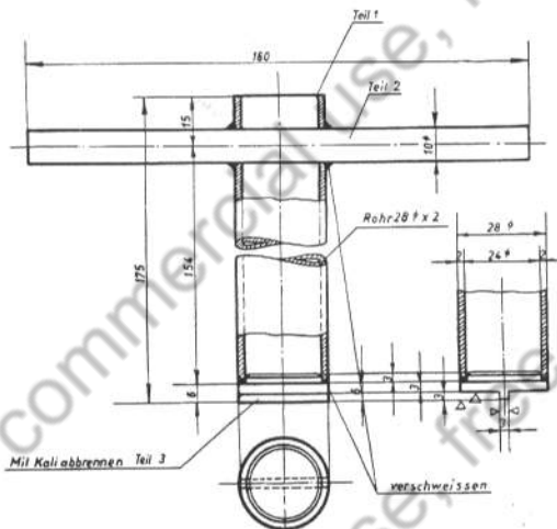
Zapfenschlüssel. Zeichn. Nr. W 212/5.
