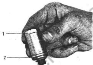
Rückschlagventil mit Schlüssel SW 22 ausschrauben.
