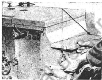
2 Renkverschlüsse öffnen (1). Deckel abnehmen.
