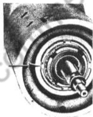
Anlasser-Scheiben-Kupplung (in Ordnung)
