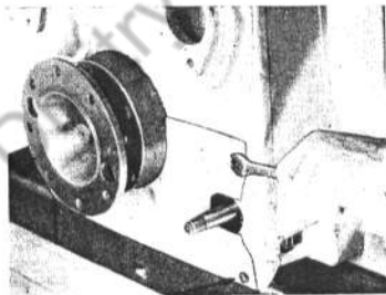
3 Schrauben mit Schlüssel SW 10 ausschrauben. Blech am Antriebsflansch abnehmen.
