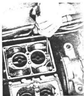
Ausgleichdüse mit Schraubenzieher ausschrauben.
