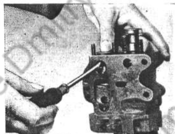
Einsatzstück in seine Bohrung einführen. Federn des Druckregelventils zusammendrücken. Einsatzstück mit Schraubenzieher festklemmen.
