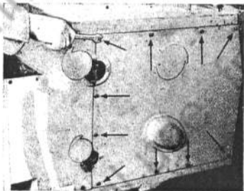
2 Schaudeckel öffnen. 12 Schrauben mit Schlüssel SW 10 ausschrauben, rechtes Seitenblech abnehmen.
