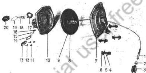
Kupplungsverzögerer zerlegt.
