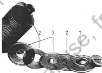
Deckel (1), Filtersiebe (2) und Filterbleche (3) abnehmen. Alle Teile mit P 3, Cehaponlösung oder dergleichen reinigen. Zusammenbau in umgekehrter Reihenfolge.
