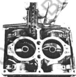
Schwimmerventil mit Schlüssel SW 17 ausschrauben.
