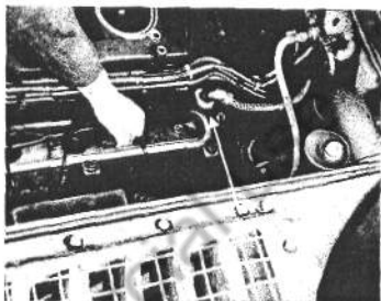
Entstörtschlauch mit Schlüssel SW 36 abschrauben.
