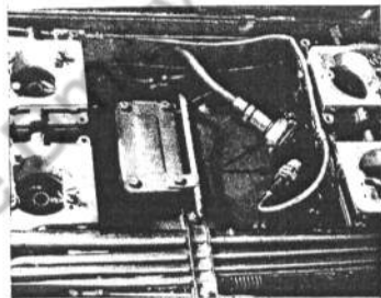
Einstellung der Düsen am hinteren Vergaser.
