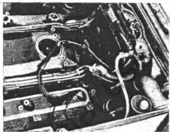
Zündleitung aus der Zylinderkopfhäube etwa 10 cm herausziehen
