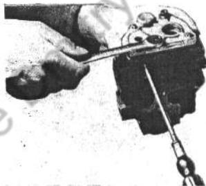
Führungsbolzen in den Deckel einfädeln. Deckel aufsetzen und festschrauben.
