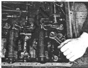
Rückschlagventil mit Schlüssel SW 22 ausschrauben.
