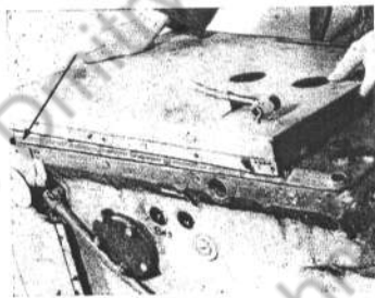
1 Schraube mit Schlüssel SW 10 ausschrauben, oberen Deckel abnehmen.
