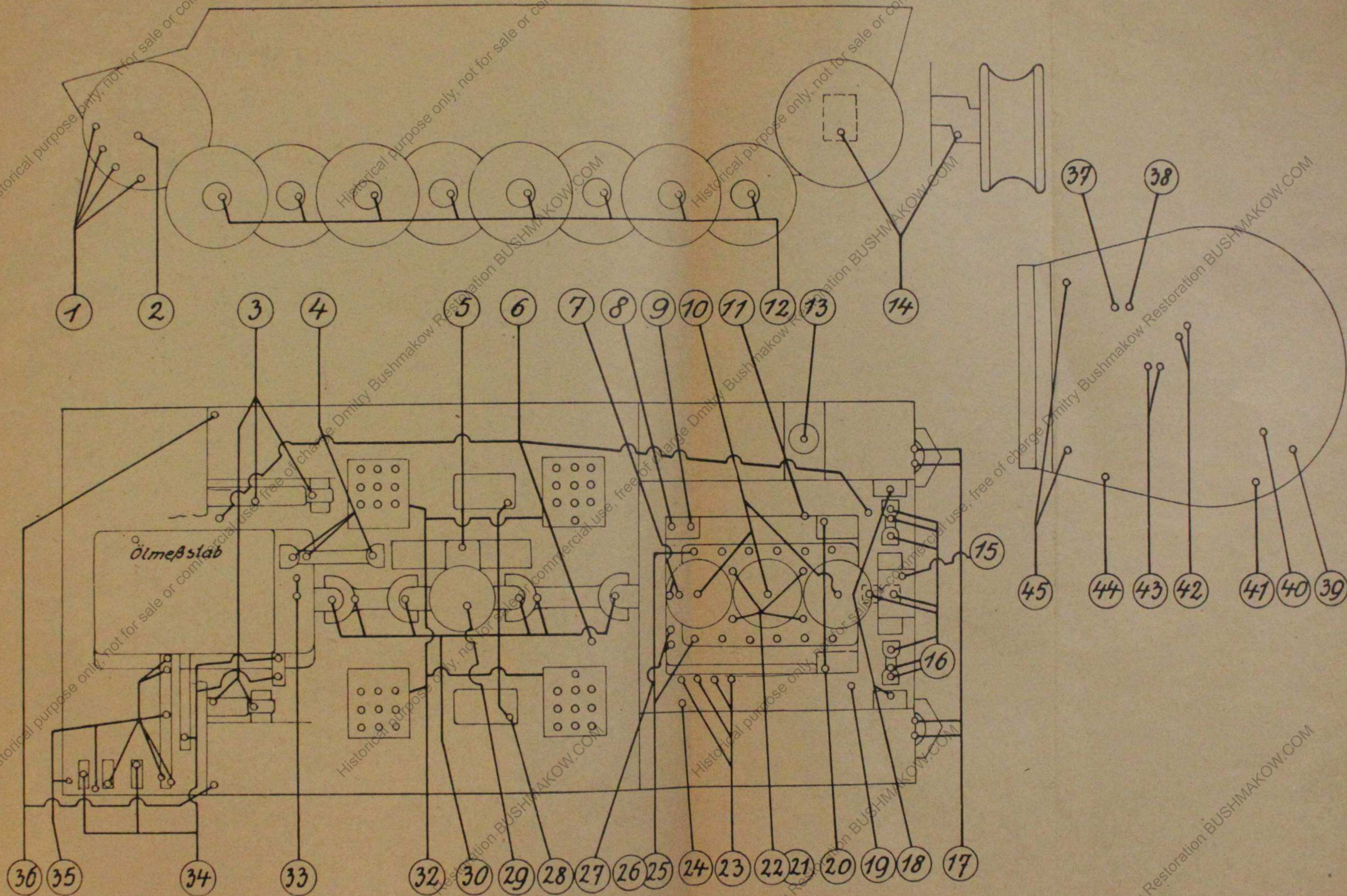
Schmierplan Pz Kpfw Tiger Ausf. E
