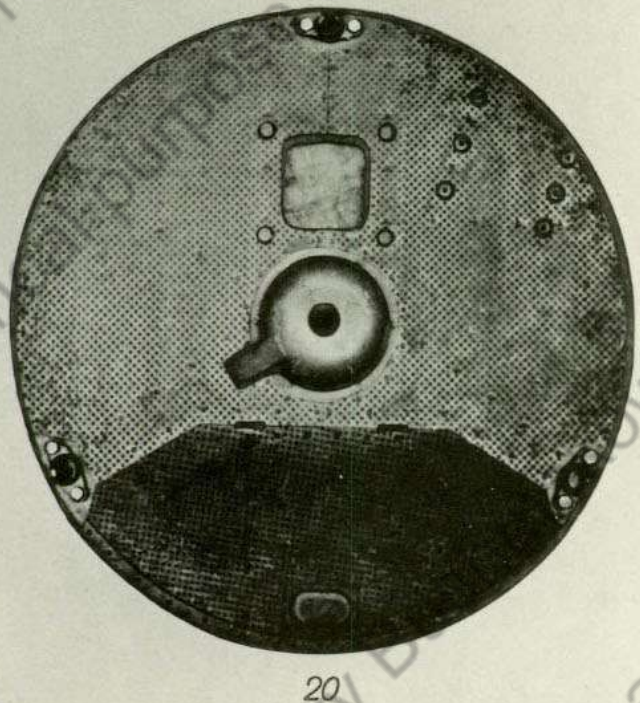
Gruppe: Drehturm [(4b) Zurrungen (Bild 1-10)] Gruppe: Drehturm [(5.) Drehbühne (Bild 11-20)]
