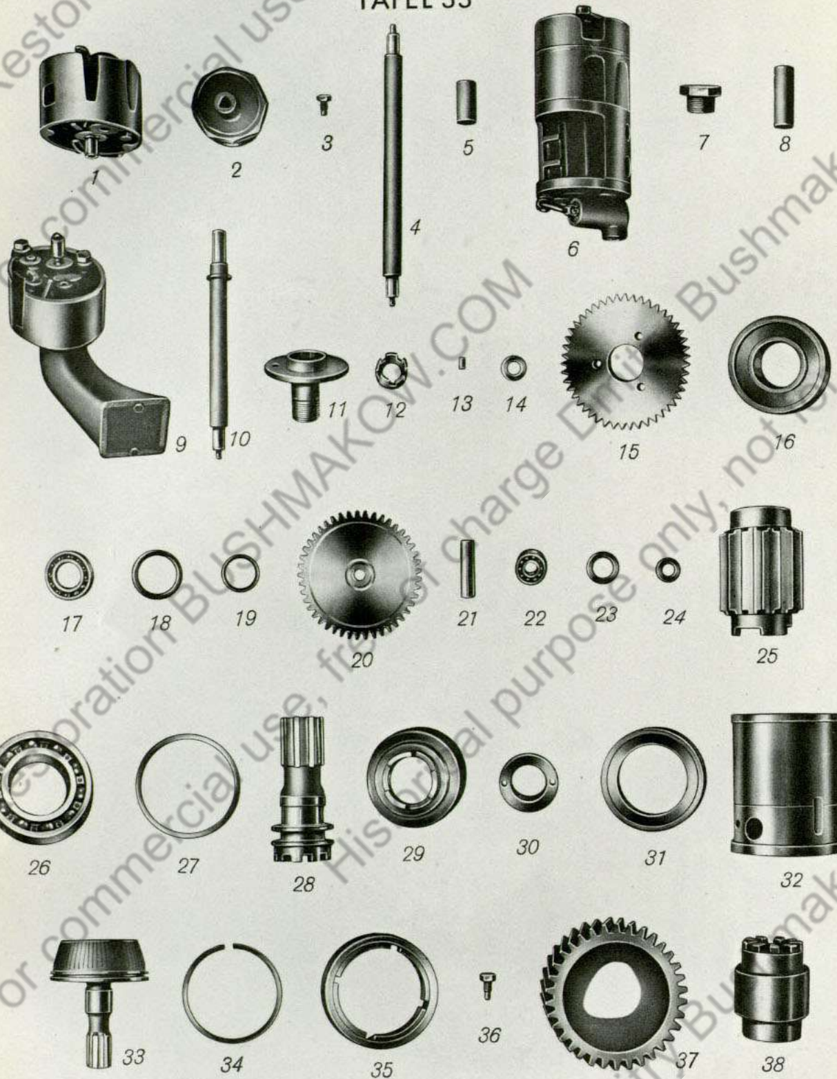
Gruppe: Schaltgetriebe mit Kupplung
