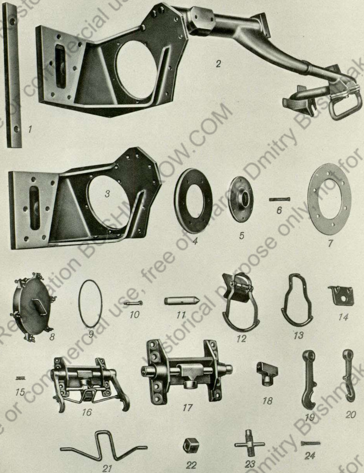
Gruppe: Drehturm [(2.) Einbauteile]
