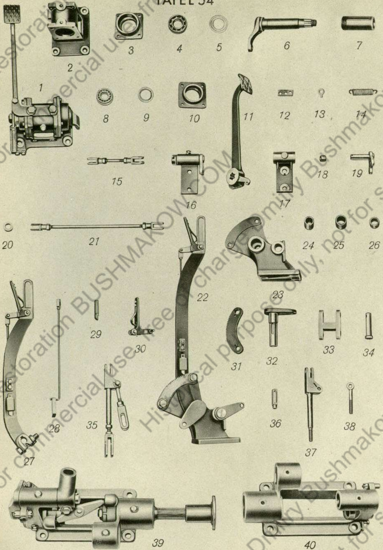
Gruppe: Hand- und Fußhebelwerk
