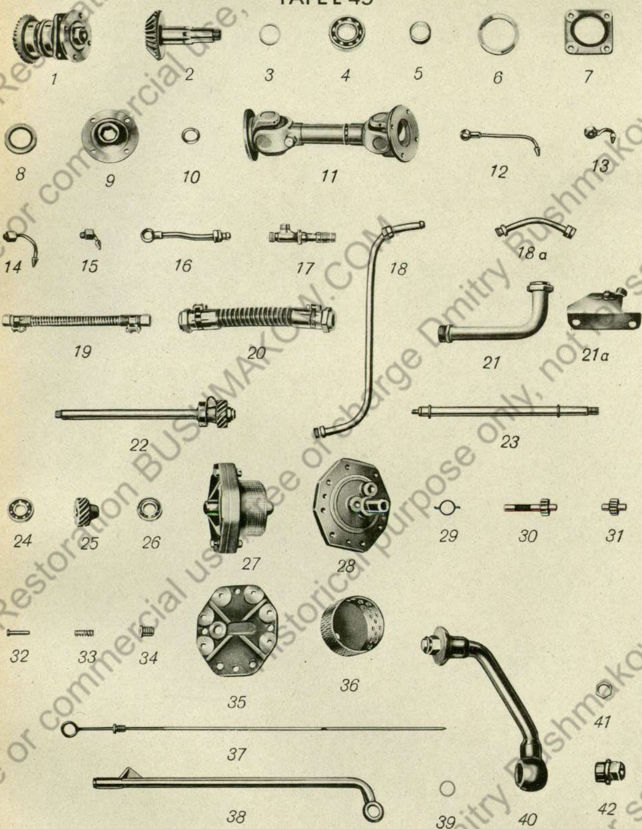
Gruppe: Antrieb für Lüfter
