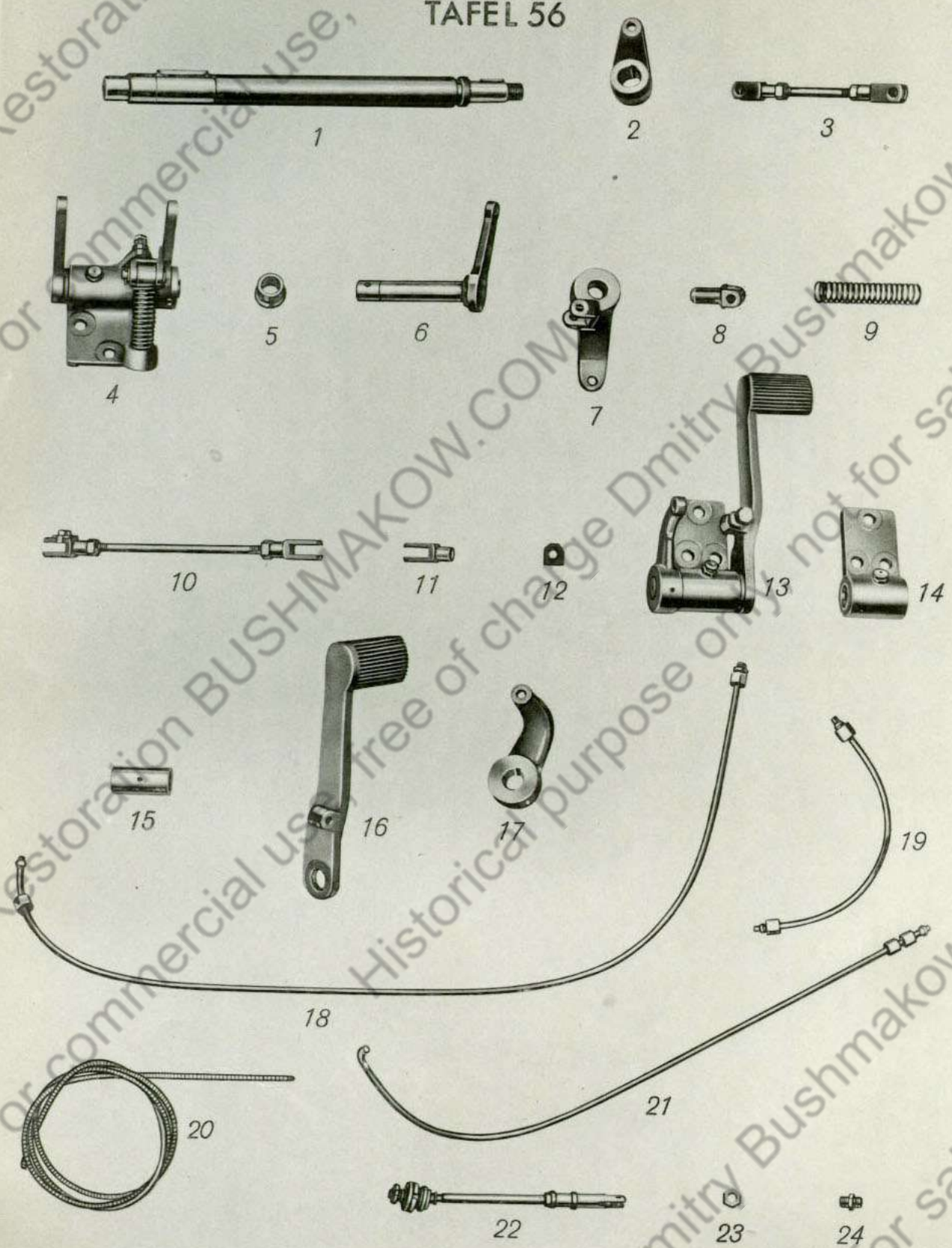
Gruppe: Hand- und Fußhebelwerk
