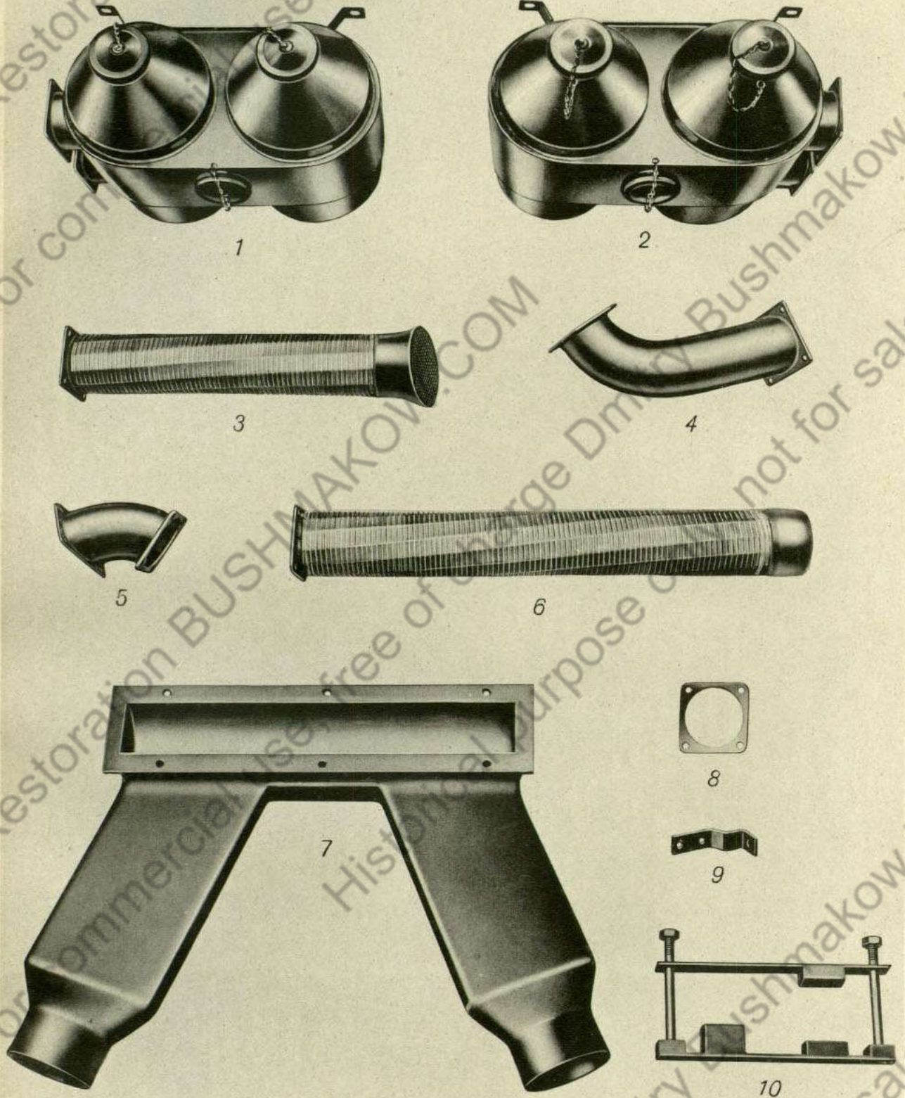
Gruppe: Kühlanlage (Wasserwirbler)
