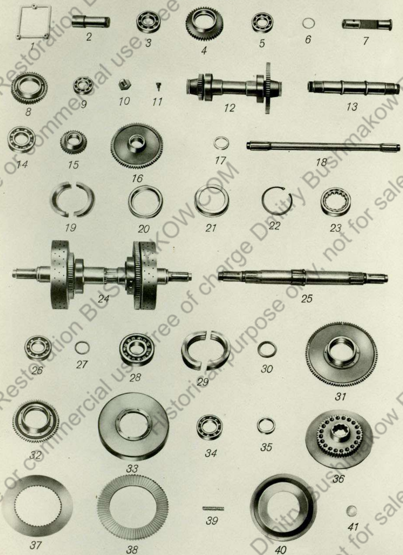
Gruppe: Lenkgetriebe
