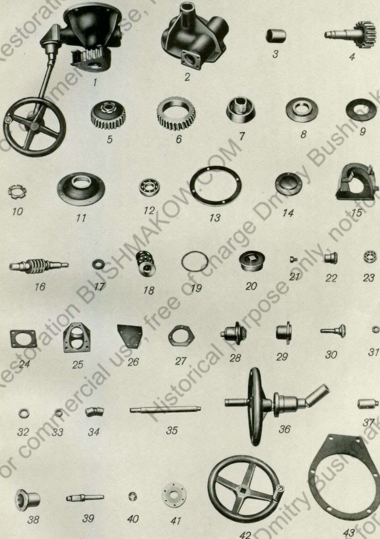
Gruppe: Höhenrichtmaschine
