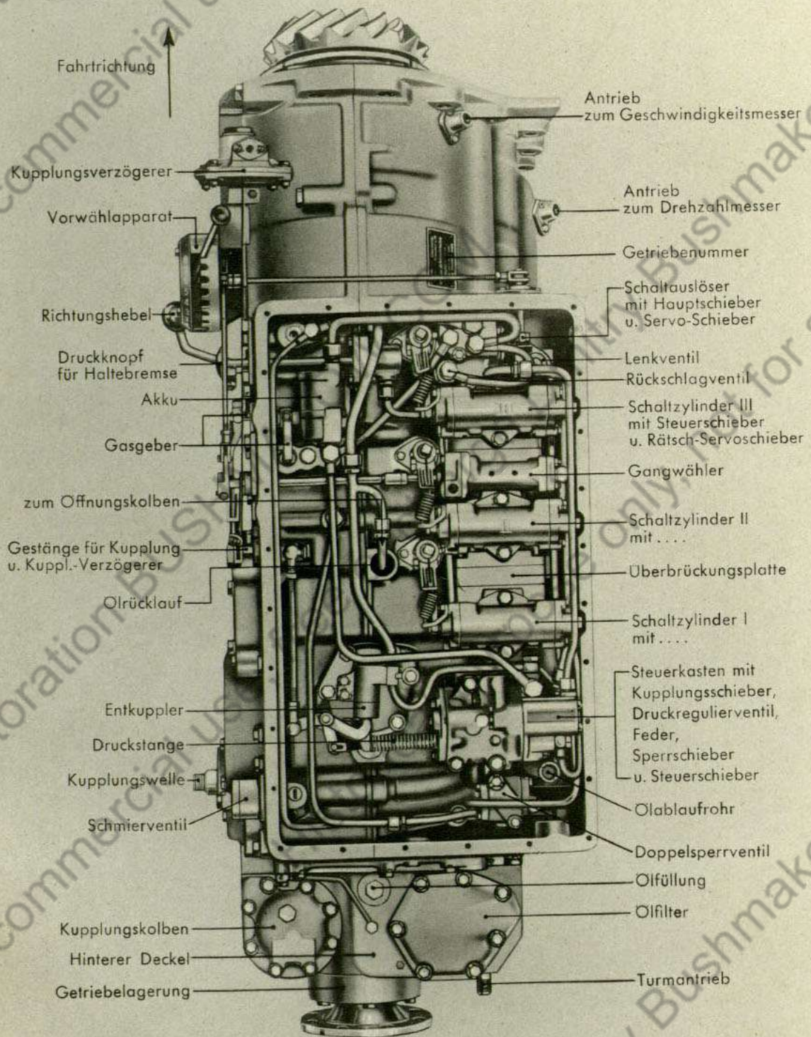
Gruppe: Schaltgetriebe mit Kupplung (Schnittbild)
