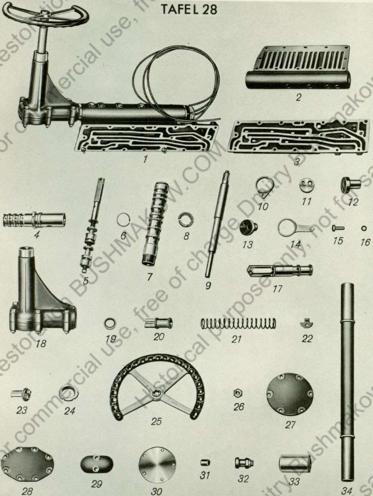
Gruppe: Lenkgetriebe
