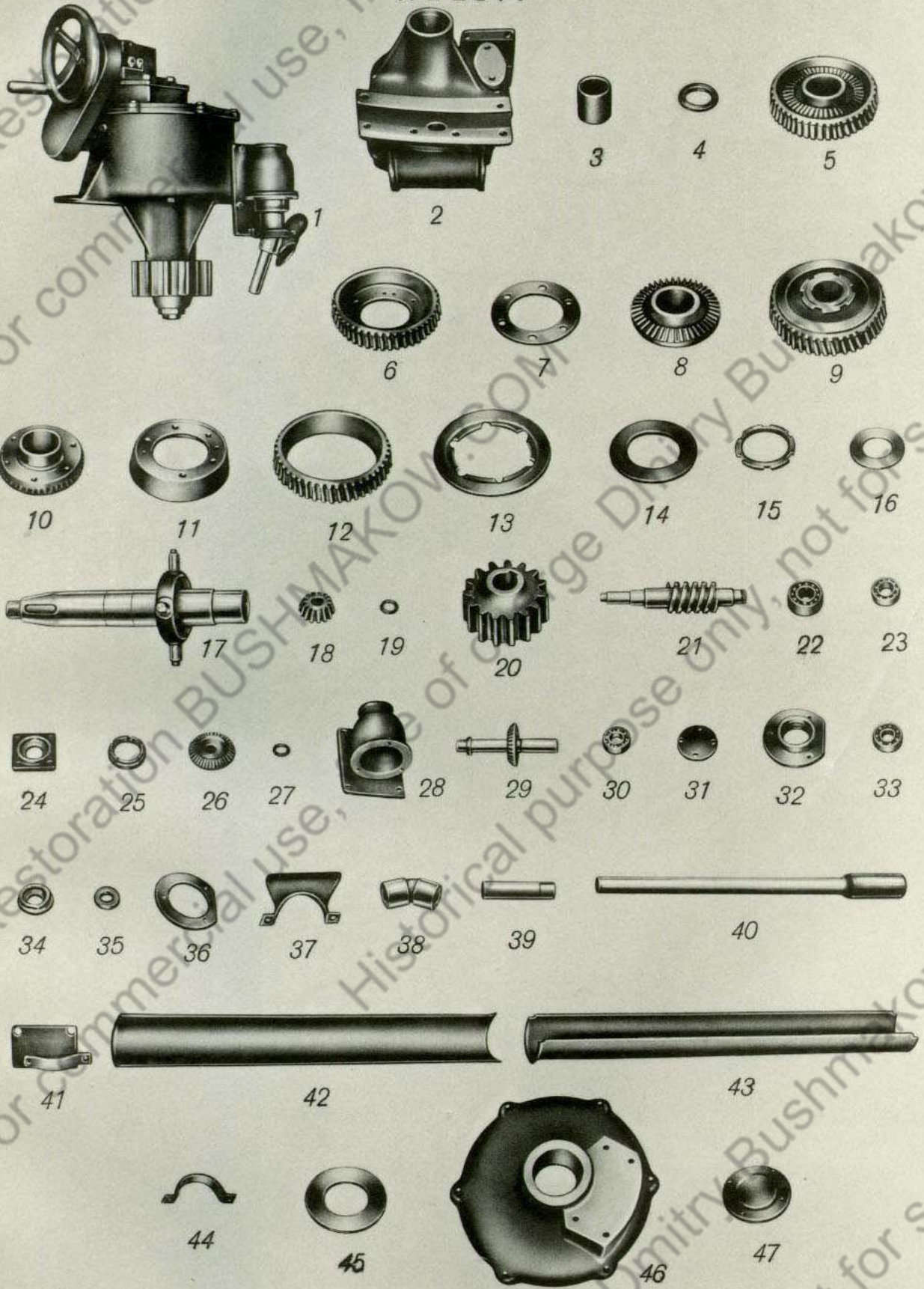
Gruppe: Turmschwenkwerk
